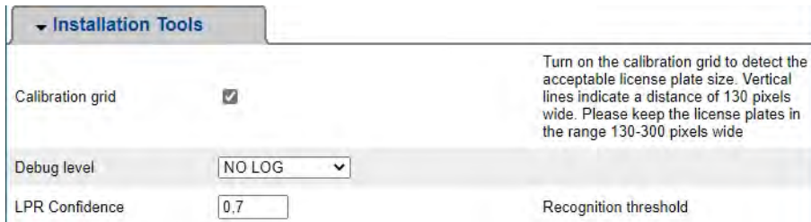
Abb. 23: Installationswerkzeuge
