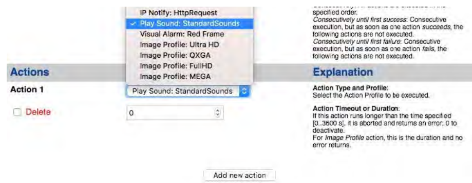
Abb. 32: Aktionstyp und Profil auswählen
