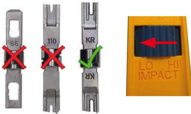
Abb. 62: Krone LSA-Plus-Anlegewerkzeug auf GERINGE Kraft eingestellt
