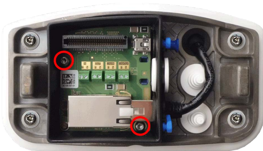
Abb. 55: Anschlussbox RJ45 (Draufsicht) mit zwei Schrauben (rot hervorgehoben) an Montageplatte montieren
