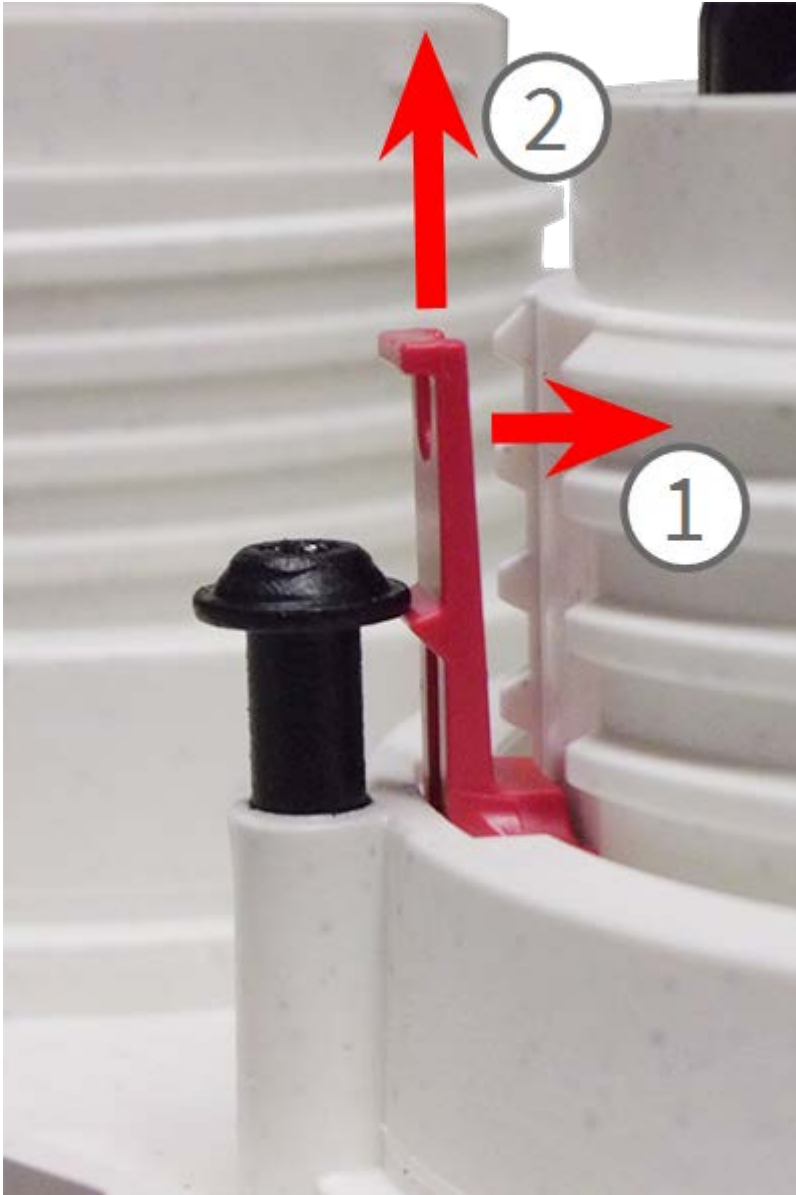
Abb. 19: Sicherungsclip entfernen
