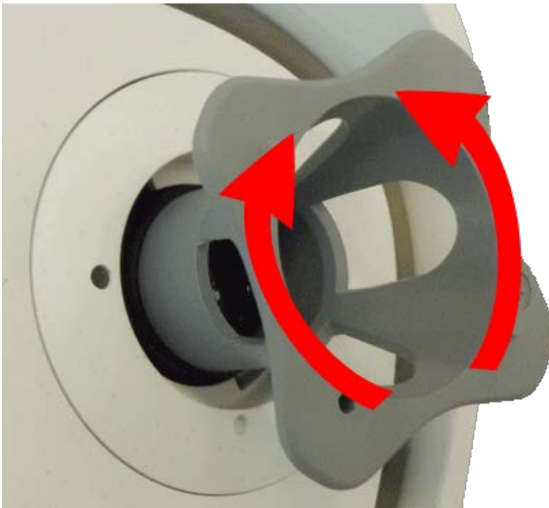
Abb. 84: Objektivfokus anpassen
