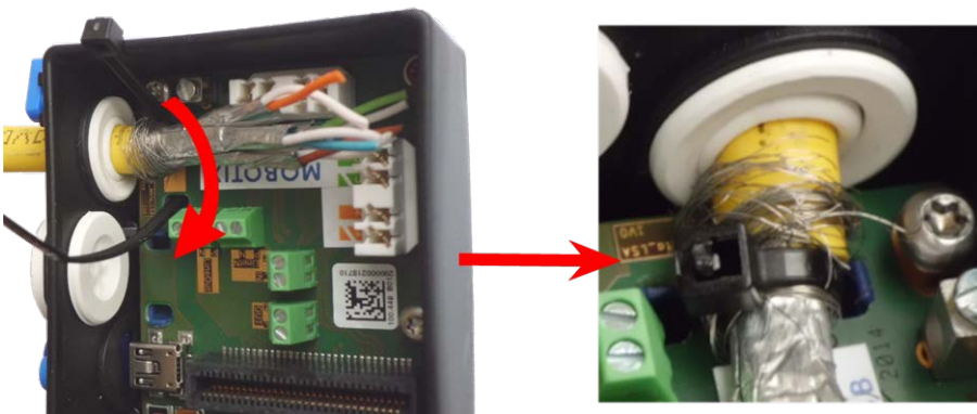
Abb. 61: Kabelbinder unter Netzkabel eingeführt
