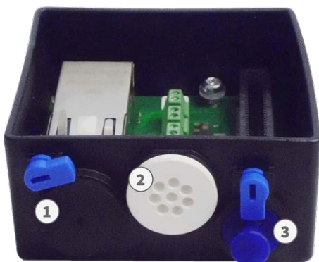
Abb. 46: Anschlussbox RJ45
