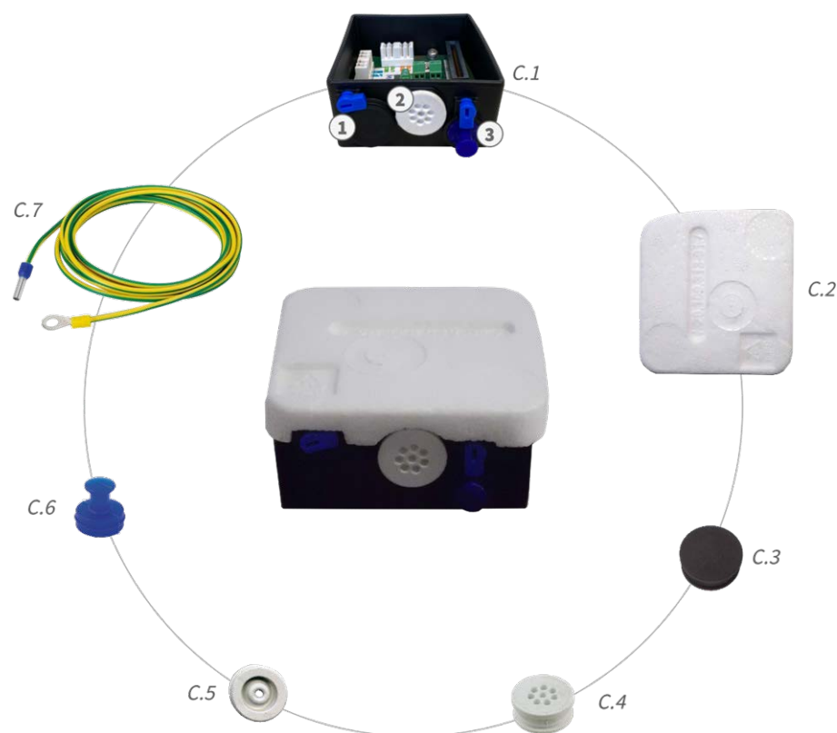
Abb. 3: Lieferumfang M73 Anschlussbox LSA
