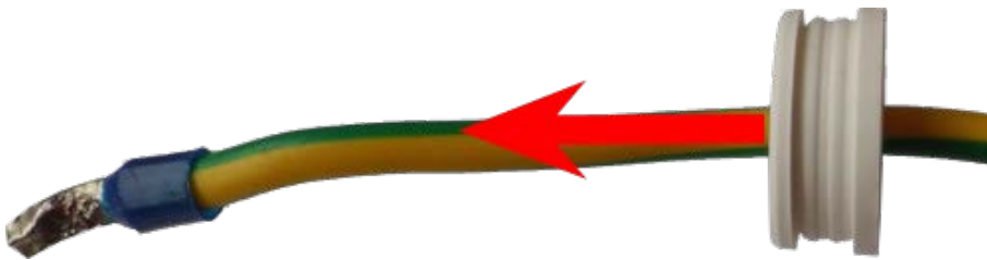
Abb. 64: Masseleitung mit einadrigem Gummistopfen C.4
