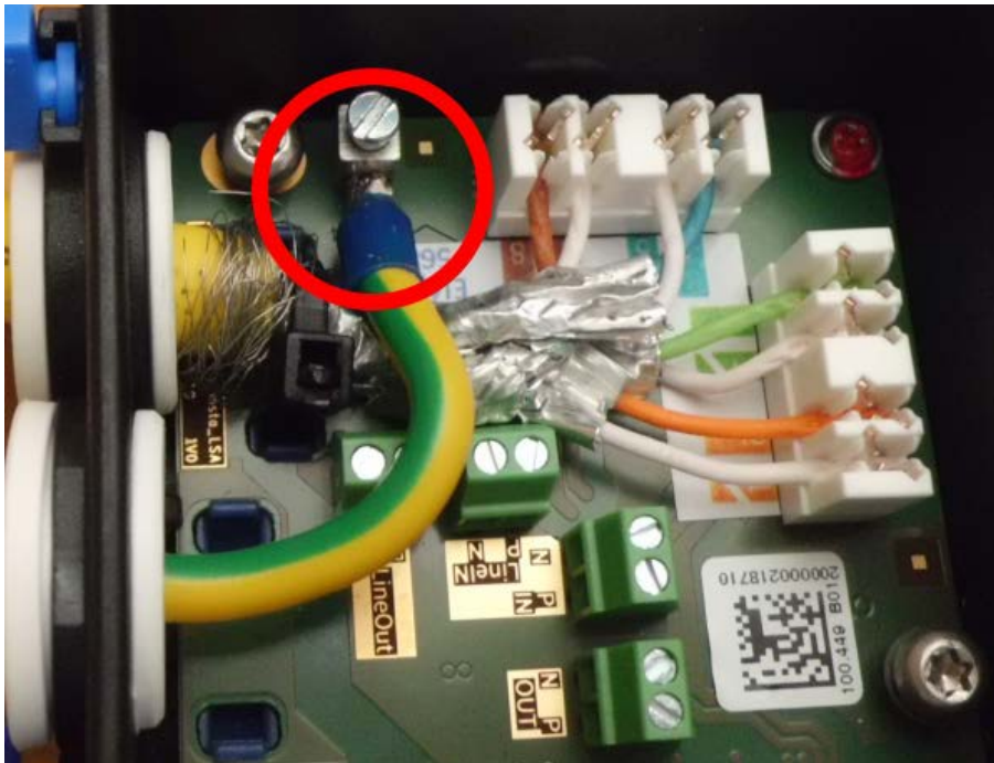
Abb. 66: Masseleitung mit Klemme verbunden
