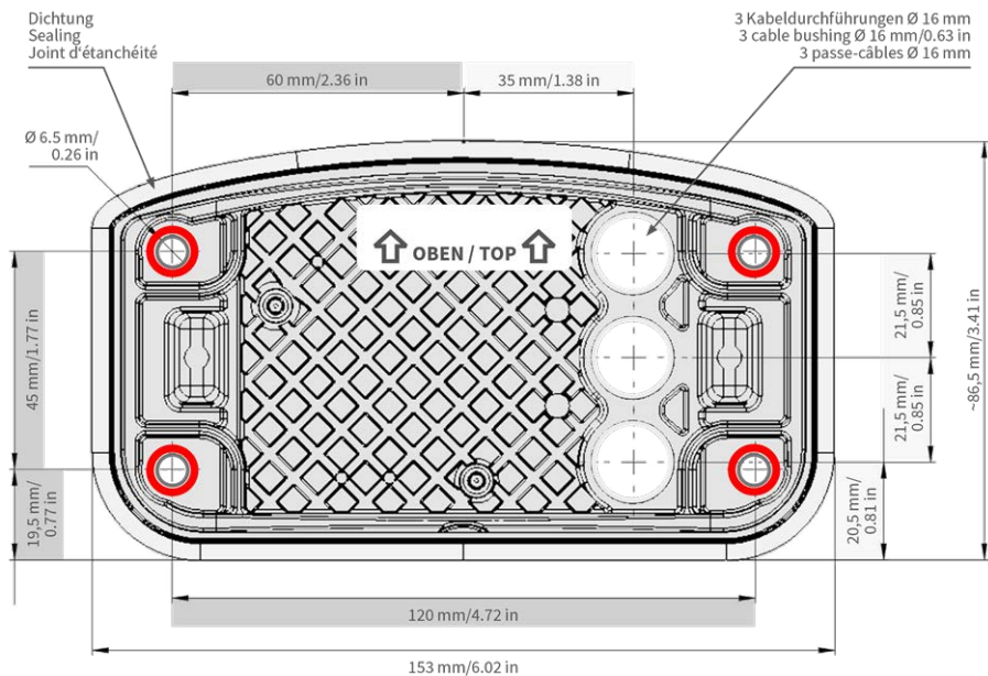
Abb. 30: Montageplatte mit Bohrungen zur Positionierung der Befestigungsschrauben
