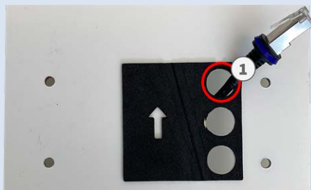
Abb. 43: Vorbereitet für Anschlussbox RJ45
