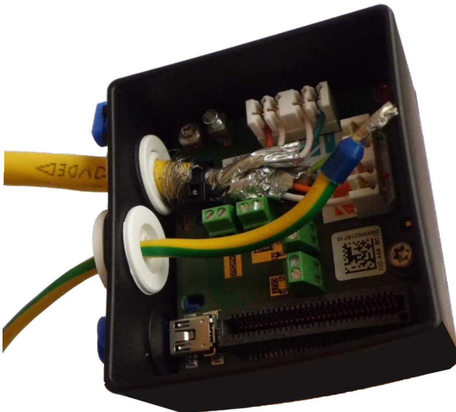
Abb. 65: Masseleitung eingesteckt, Stopfen richtig eingesetzt
