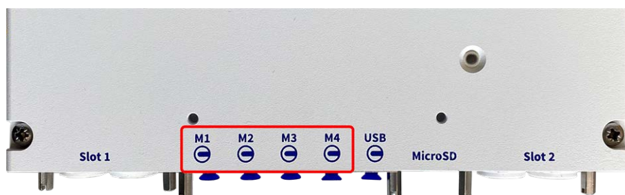
Fig. 22: Connecteurs de modules de la S74
