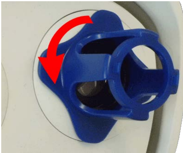
Fig. 33: Tournez le module de capteur à fond dans le sens inverse des aiguilles d'une montre
