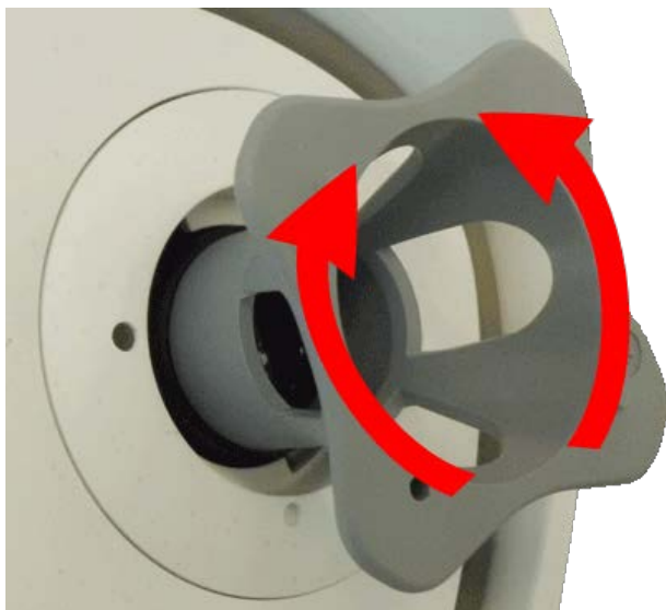
Fig. 34: Réglage de la mise au point de l'objectif
