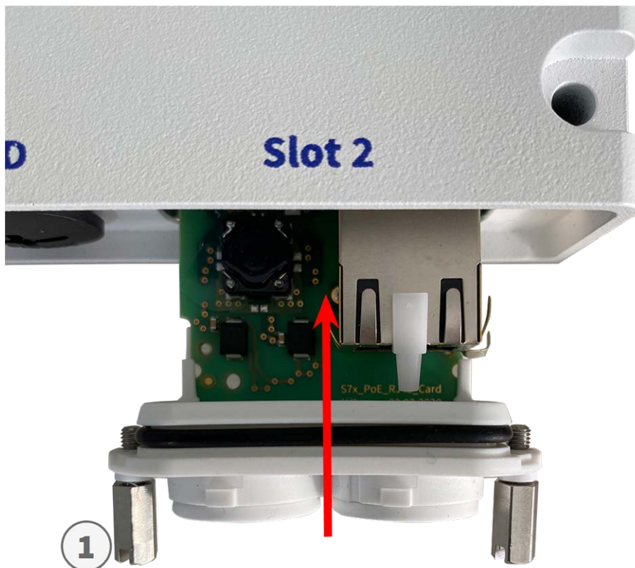
Fig. 19: Connexion de la carte d'interface RJ45
