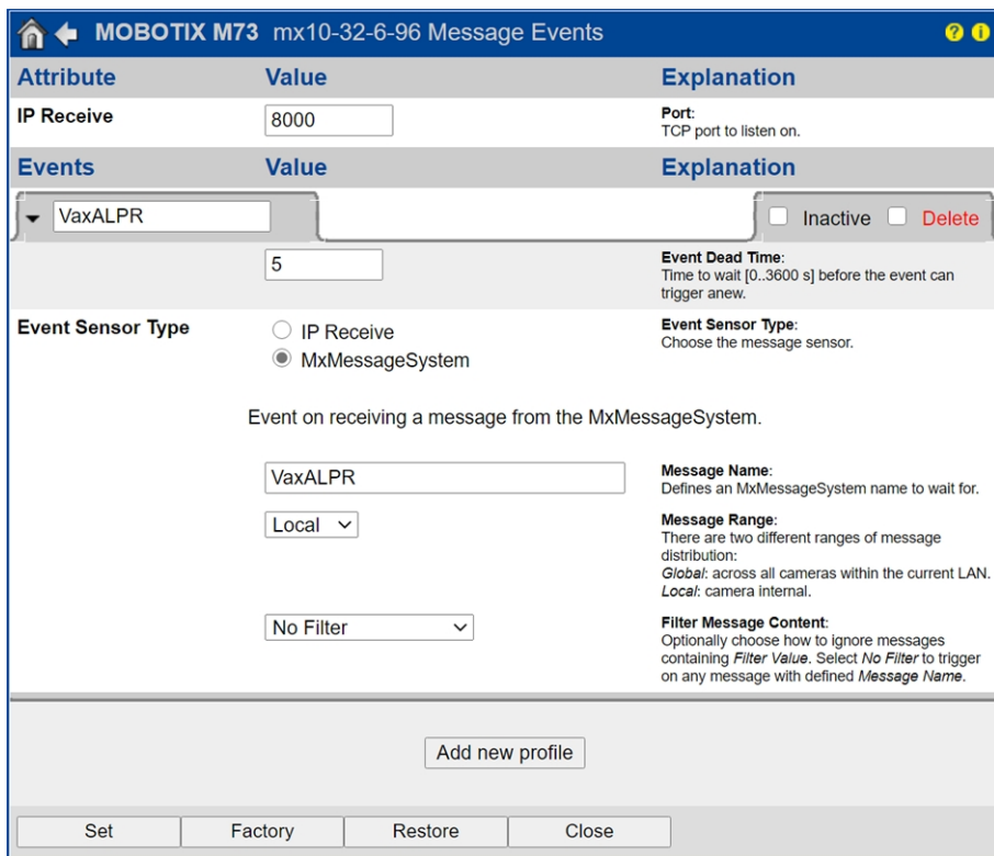
Abb. 29: Beispiel: Generisches Nachrichtenergebnis von VAXTOR License Plate Recognition App
