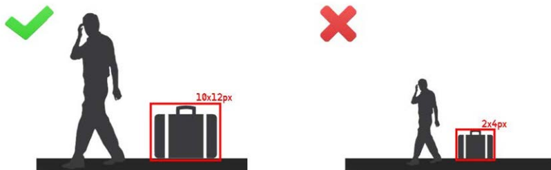
AI-LOST – Zielgröße
