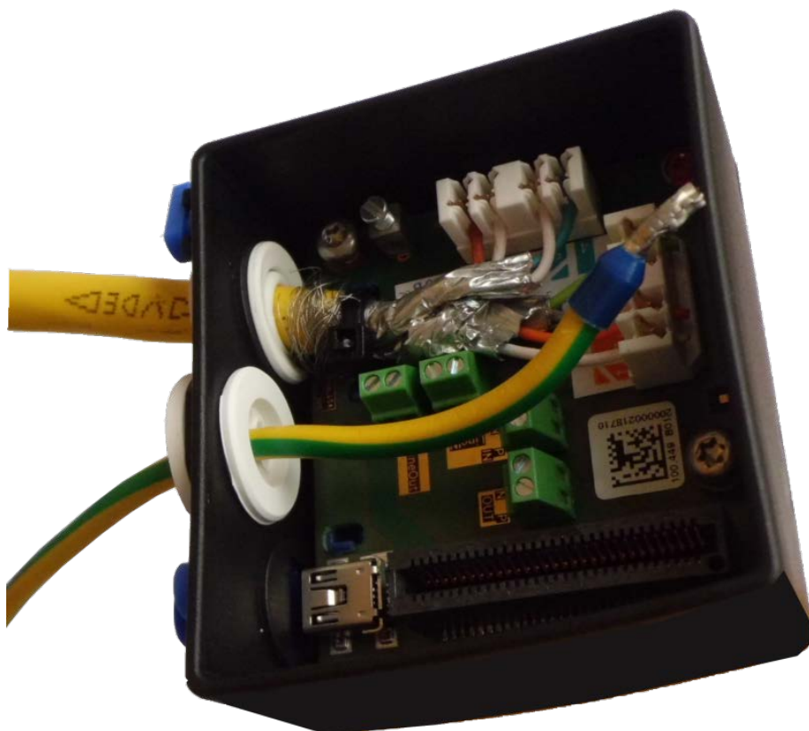
Fig. 65: Filo di massa inserito, tappo posizionato correttamente
