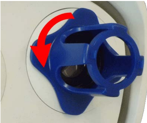
Abb. 33: Das Sensormodul bis zum Anschlag gegen den Uhrzeigersinn drehen
