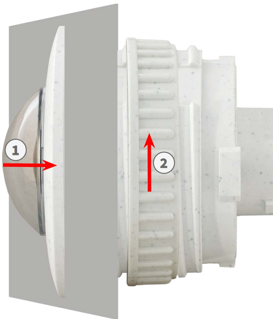
Abb. 10: Sensormodul montieren
