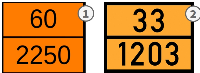
Abb. 17: Nicht konformes ADR Kennzeichen①, Konformes ADR Kennzeichen②
