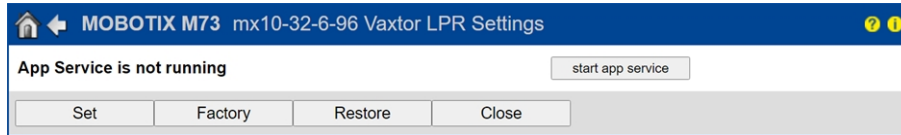
Abb. 19: Starten des App-Dienstes
