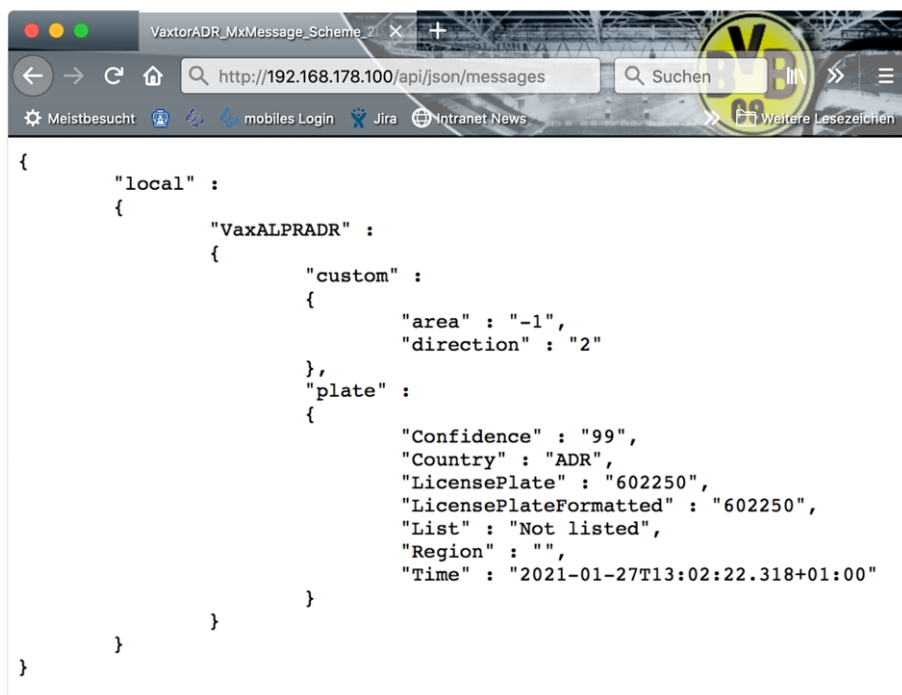
Abb. 35: Beispiel: Metadaten, die innerhalb einer MxMessage von Vaxtor License Plate Recognition / Dangerous Goods App übertragen werden
