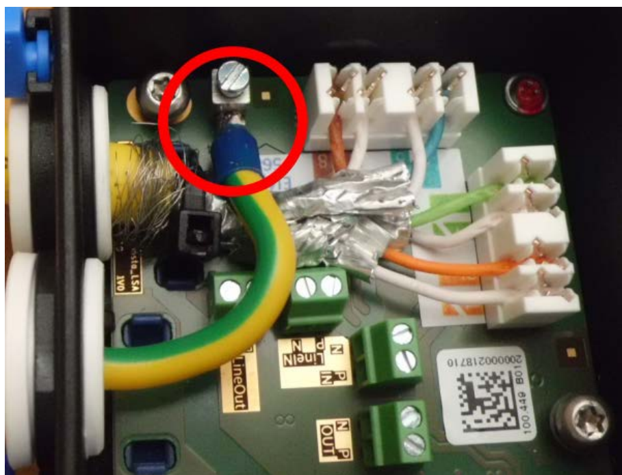
Fig. 66: Filo di massa collegato al morsetto
