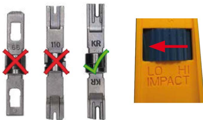
Fig. 62: Strumento LSA+/Krone impostato su impatto LOW (basso)
