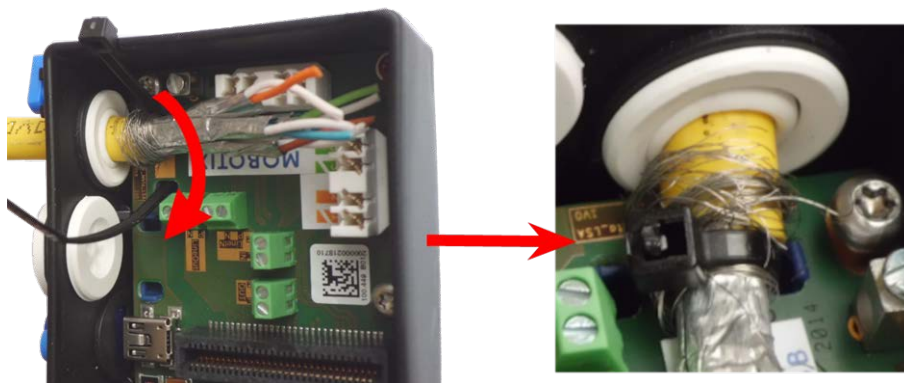
Fig. 61: Fascetta serracavi inserita sotto il cavo di rete
