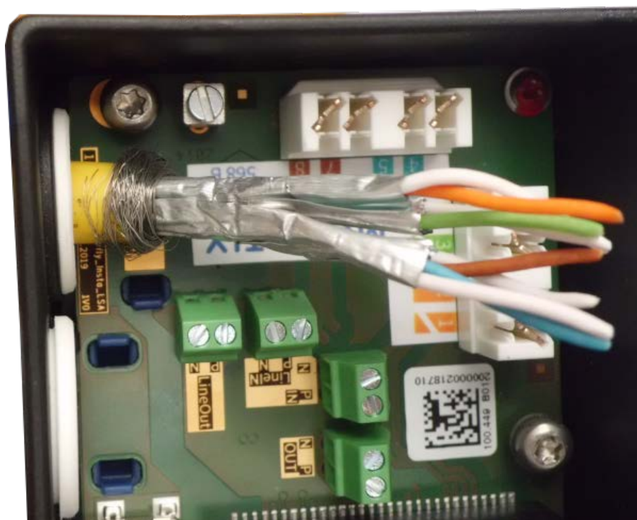
Fig. 60: Cavo di rete inserito, tappo posizionato correttamente
