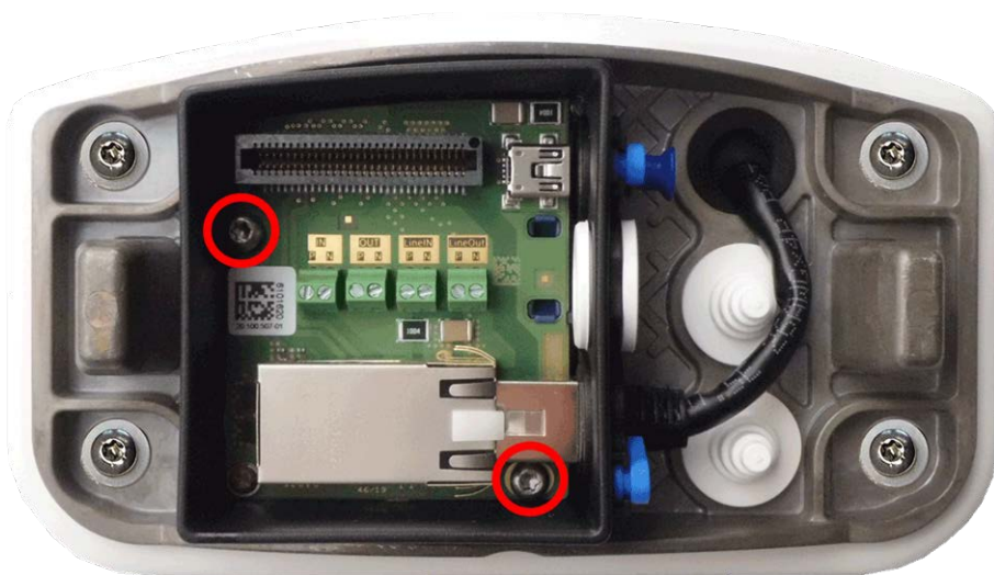
Fig. 55: Montare la Connector Box RJ45 (vista dall'alto) utilizzando le due viti (evidenziate in rosso nella figura) sulla piastra di montaggio
