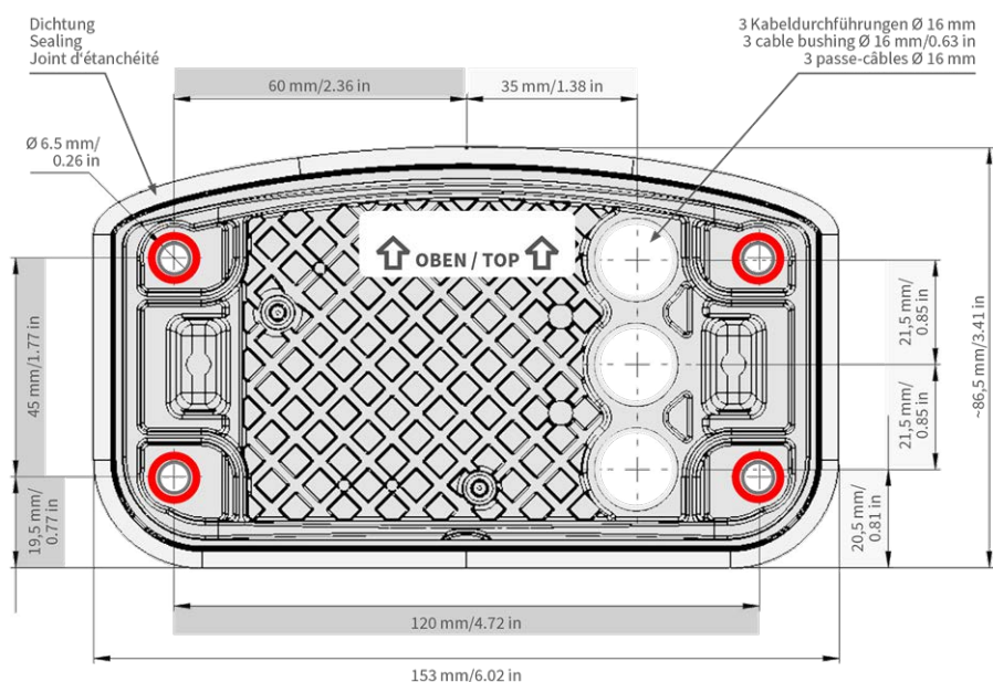
Fig. 30: Piastra di montaggio con fori per il posizionamento delle viti di fissaggio
