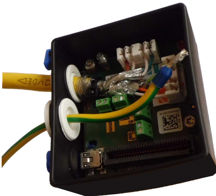
Fig. 65: Filo di massa inserito, tappo posizionato correttamente
