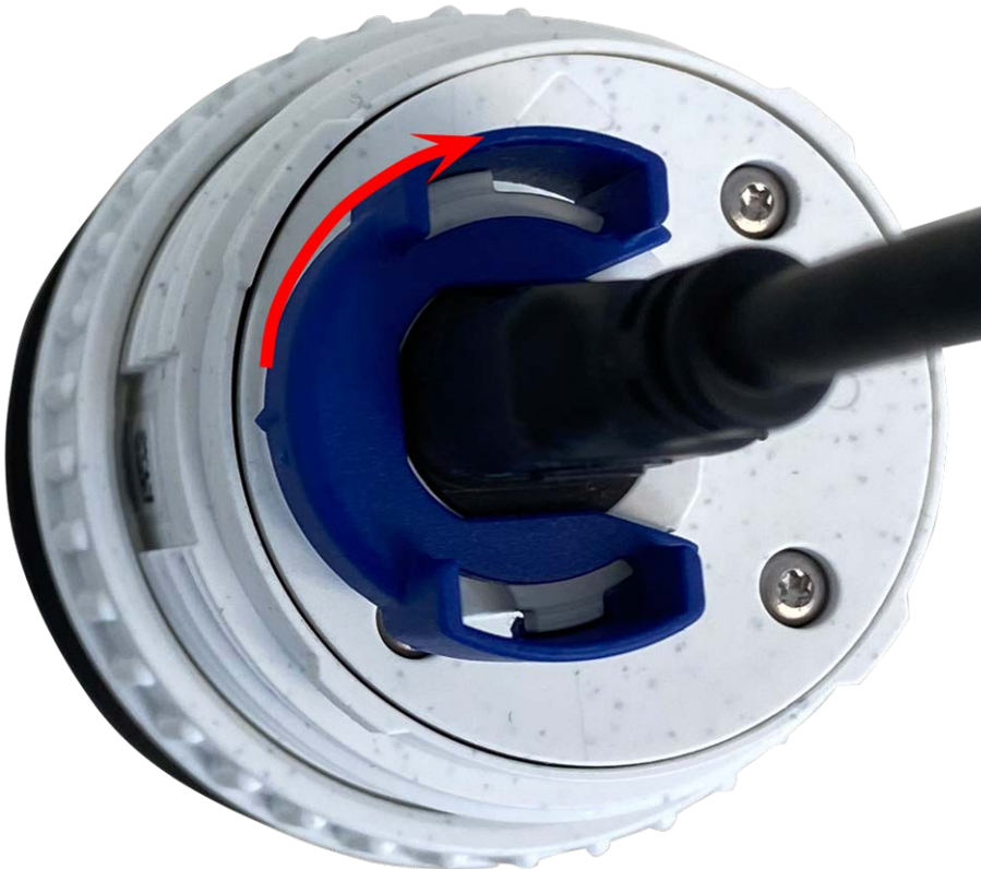
Fig. 12: Lock sensor module cable
