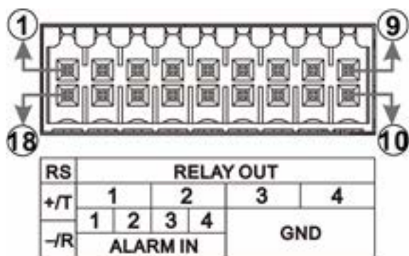
Fig. 1: Esquema de numeración de pines de los conectores E/S de alarma del MOVE NVR-8
