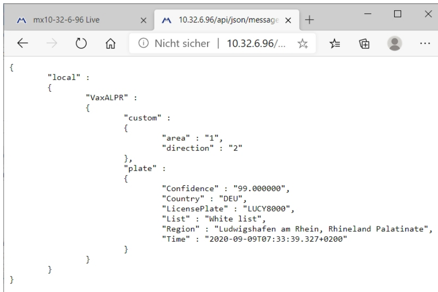
Abb. 28: Beispiel: Metadaten, die innerhalb einer MxMessage von VAXTOR License Plate Recognition App übertragen werden
