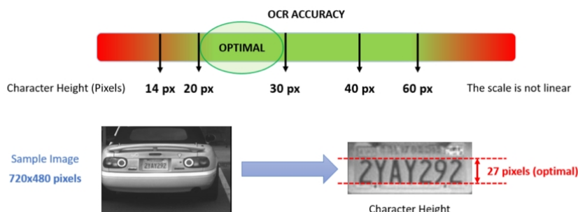
Abb. 9: Minimale Zeichenhöhe
