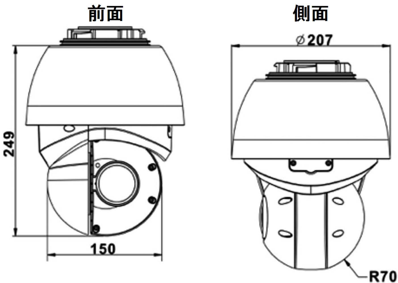
図1: MOBOTIX MOVE SpeedDome: すべての測定値の単位はmm
