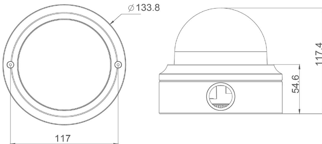
図1: MOBOTIX MOVE VandalDome: すべての測定値の単位はmm
