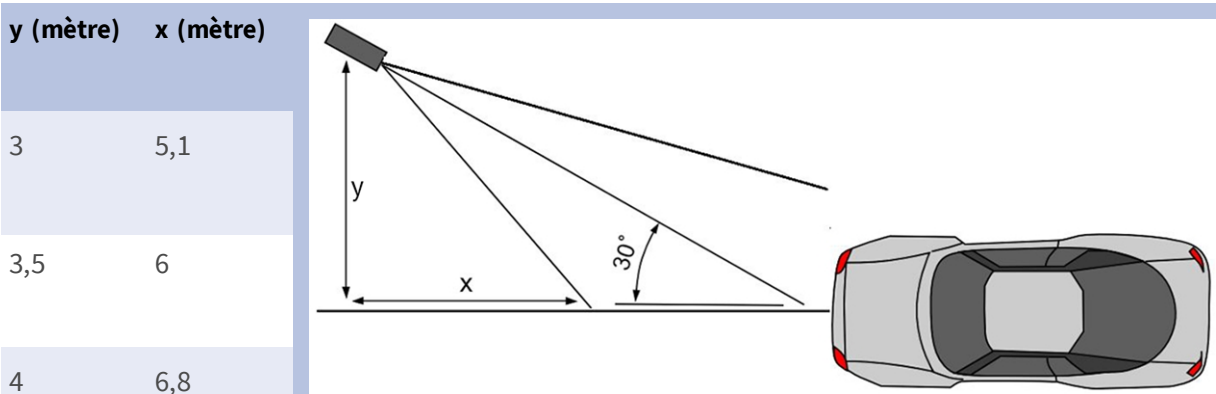
Fig. 10: Alignement horizontal de la caméra
