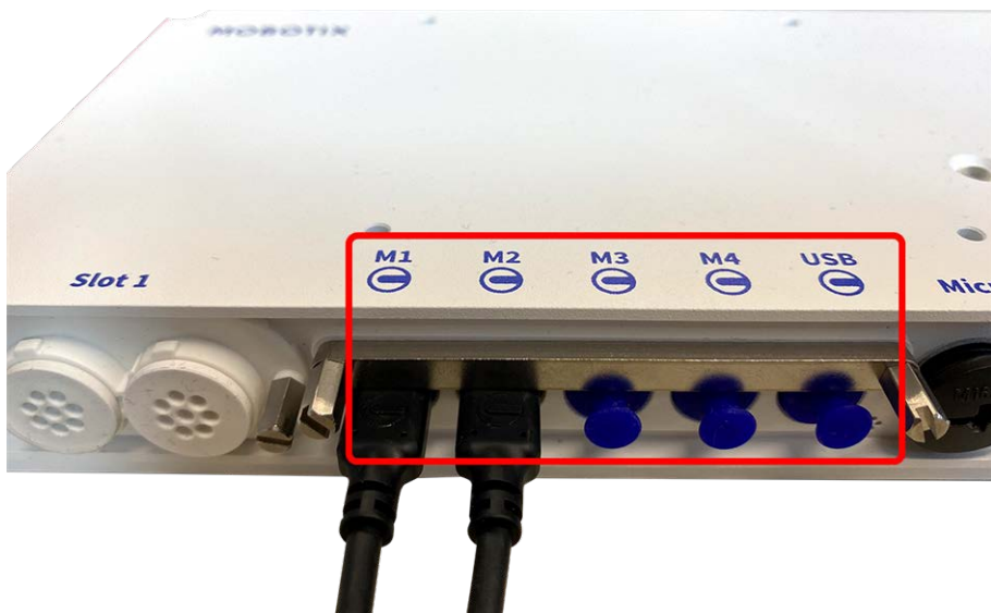
Fig. 32: 4 puertos de conexión de módulos y 1 interfaz USB-C
