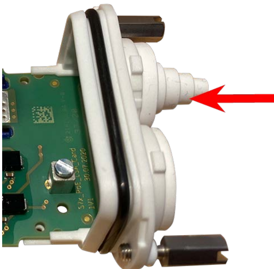
Fig. 22: Retire la cubierta de la ranura de la tarjeta de interfaz
