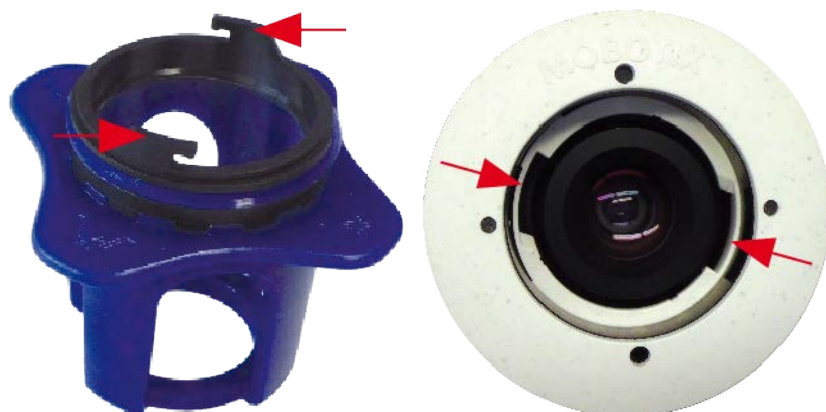
Fig. 47: Inserte el cristal de protección del objetivo con la llave de objetivo
