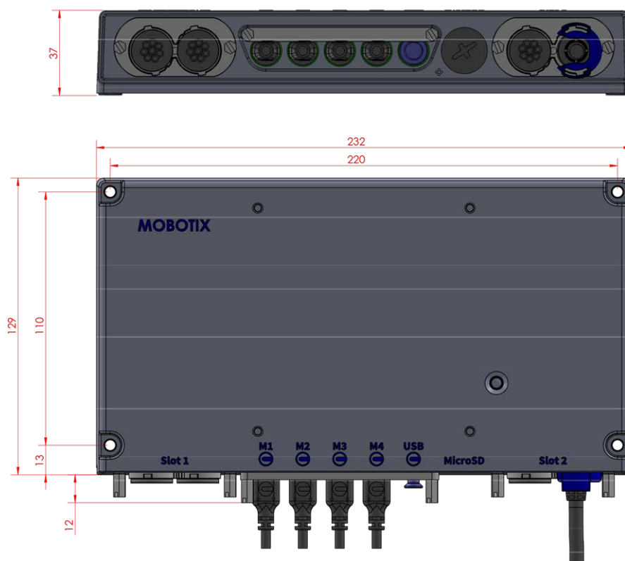
Abb. 1: S74: Alle Maßangaben in mm
