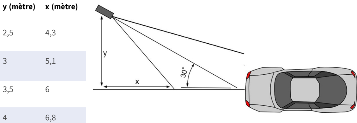
Fig. 10: Alignement horizontal de la caméra
