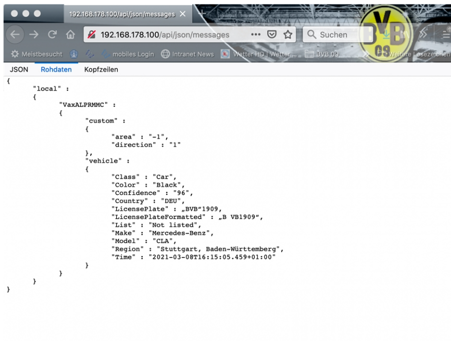
Fig. 27: Esempio: metadati trasmessi all'interno di un MxMessage dell'applicazione Vaxtor LPR & MMCR App
