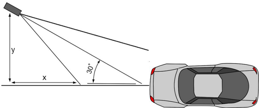
Fig. 12: Alineación horizontal de la cámara
