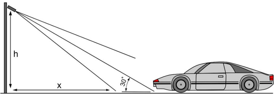
Fig. 11: Orientación vertical de la cámara
