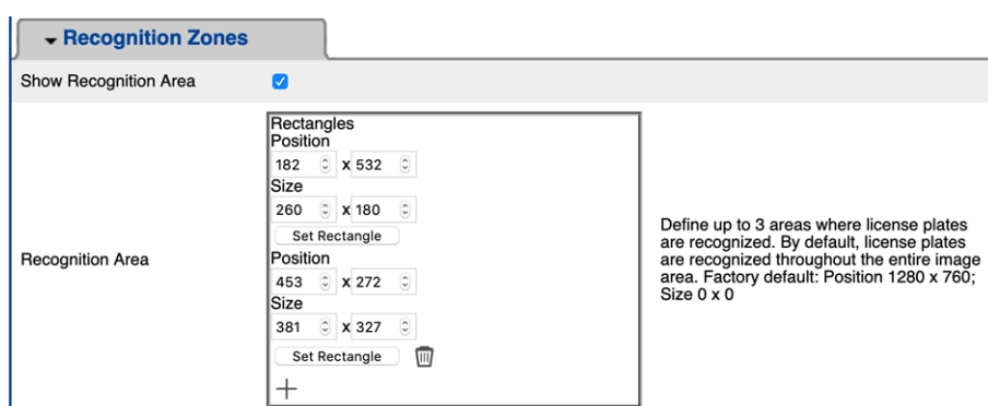
Fig. 21: Áreas de reconocimiento
