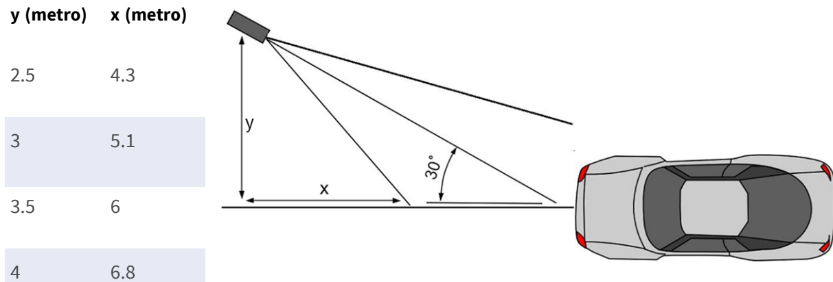
Fig. 12: Alineación horizontal de la cámara
