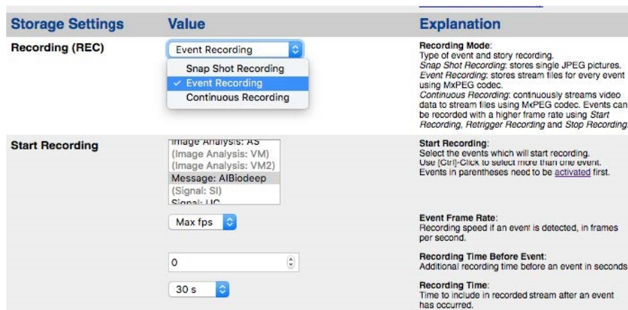
Fig. 30: Configuración de los ajustes de grabación de la cámara
