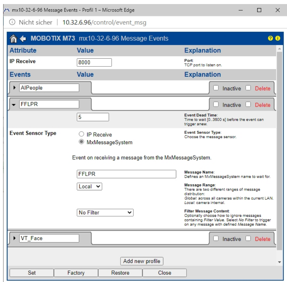
Fig. 26: Ejemplo: evento de mensaje genérico de la FF Group License Plate Recognition App - Region EUCA
