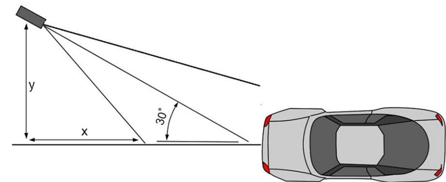
Fig. 10: Allineamento orizzontale della telecamera
