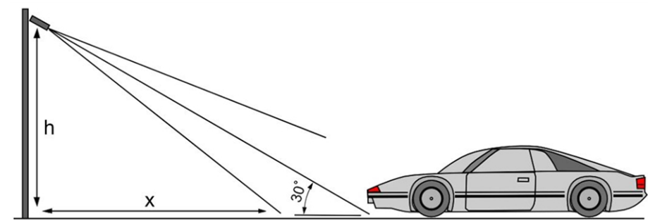
Fig. 9: Puntamento verticale della telecamera
