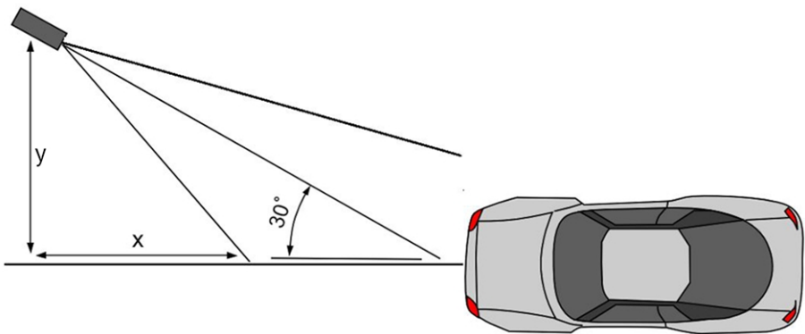
Fig. 12: Horizontale Ausrichtung der Kamera
