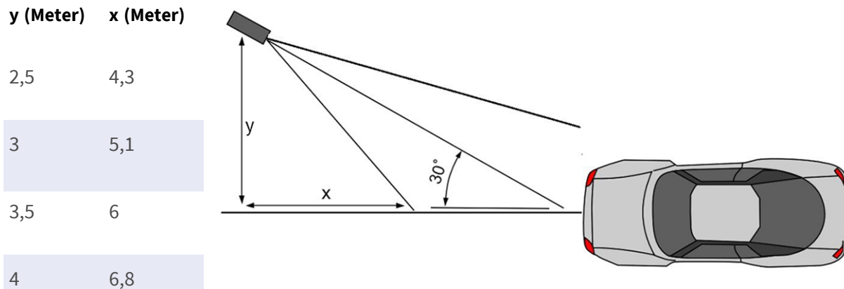
Fig. 12: Horizontale Ausrichtung der Kamera
