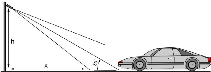
Fig. 11: Vertikale Ausrichtung der Kamera
