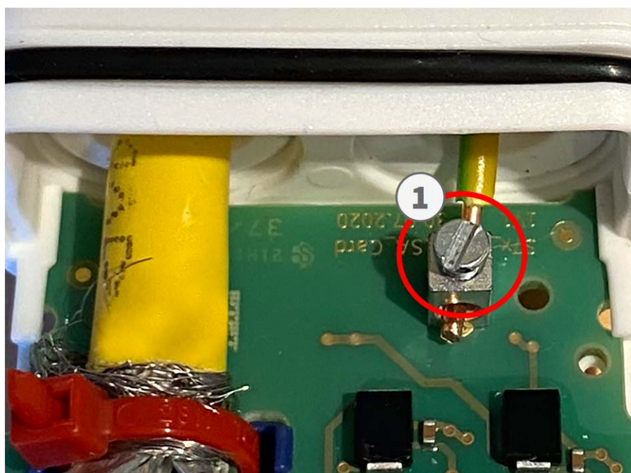
Fig. 29: Fil de terre connecté à la borne
