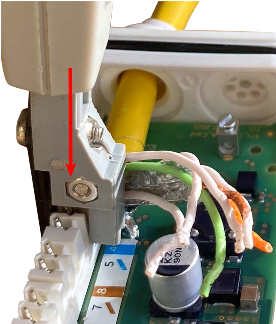
Fig. 26: Fils réseau connectés à l'aide de l'outil LSA+/Krone
