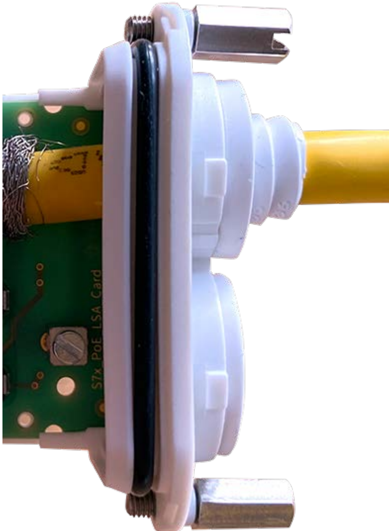
Fig. 23: Câble réseau inséré, bouchon correctement installé
