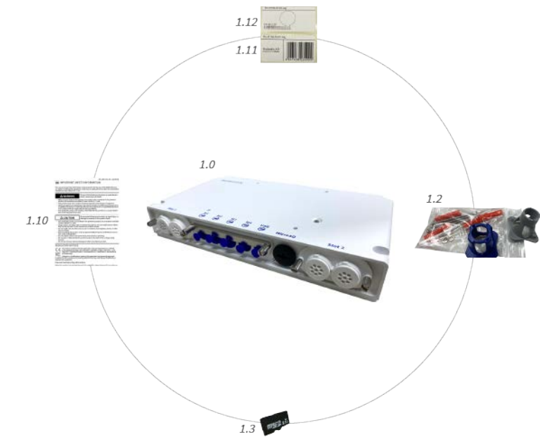
Fig. 1: Contenu de la livraison S74
