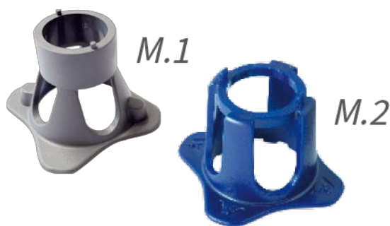
Fig. 43: Clé de montage de module M.1 et clé de montage d'objectif M.2 de la S74
