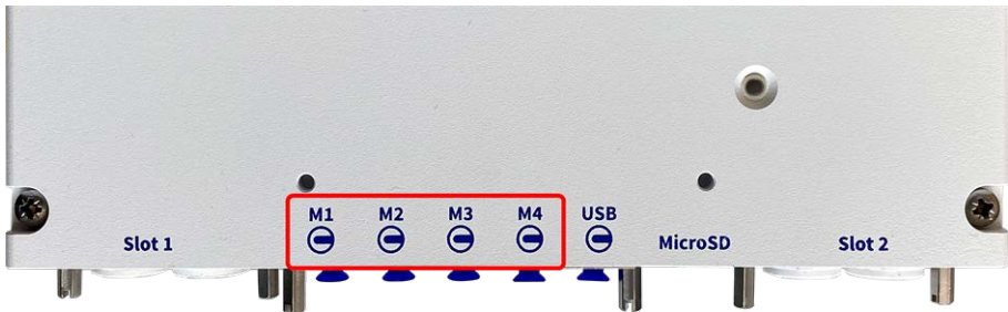
Fig. 33: Connecteurs de modules de la S74
