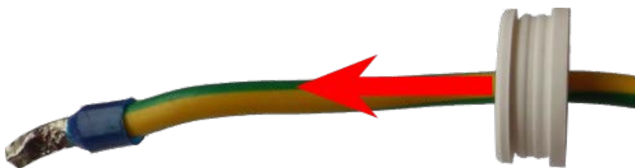
Fig. 27: Fil de terre avec bouchon en caoutchouc à un fil
