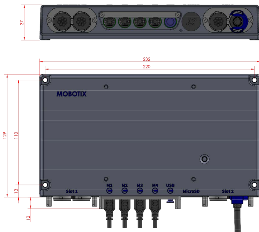
Fig. 5: S74 : toutes les mesures sont en mm
