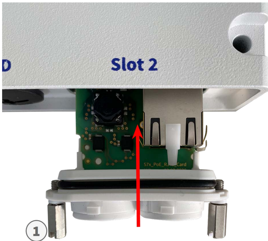
Fig. 19: Connexion du Carte d'interface RJ45
