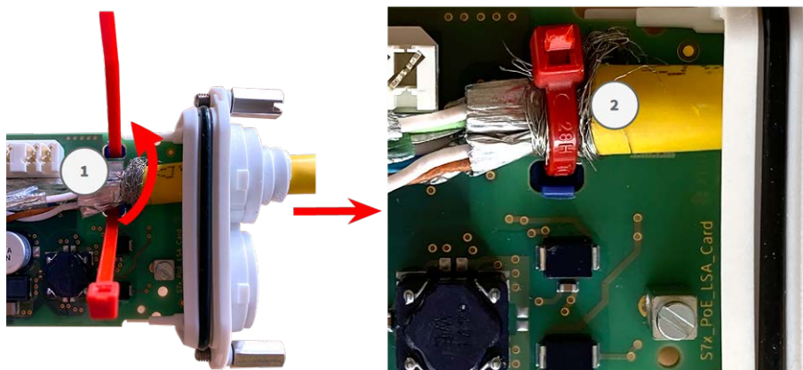
Fig. 24: Serre-câble inséré sous le câble réseau
