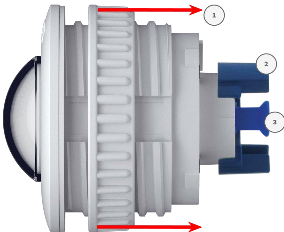
Fig. 9: Preparazione del modulo sensore per il montaggio
