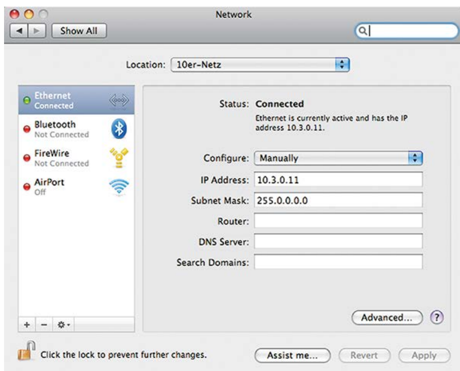
Fig. 39: Impostazioni di rete su macchine MacOS
