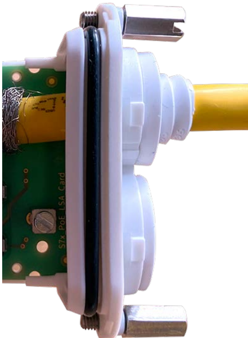
Fig. 23: Cavo di rete inserito, tappo posizionato correttamente
