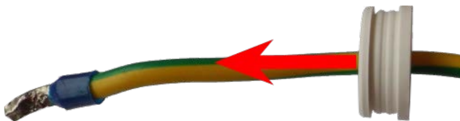
Fig. 27: Filo di massa con tappo in gomma a filo singolo
