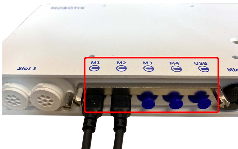
Fig. 32: 4 porte per connettore modulo e 1 interfaccia USB-C
