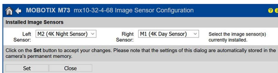
Fig. 50: Configurazione dei moduli sensore
