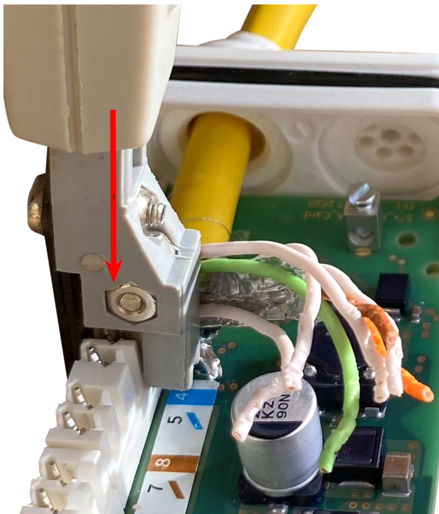
Fig. 26: Fili del cavo di rete collegati mediante lo strumento LSA+/Krone
