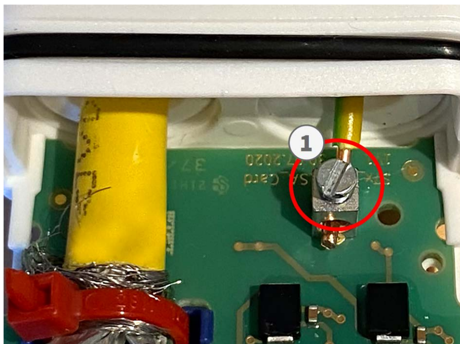
Fig. 29: Filo di massa collegato al morsetto
