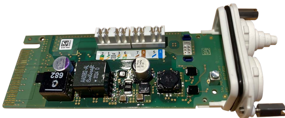
Fig. 20: Scheda di interfaccia LSA
