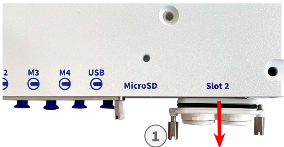
Fig. 18: Rimuovere il coperchio dallo slot della scheda di interfaccia
