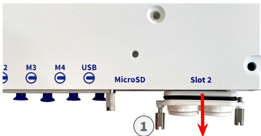
Fig. 22: Rimuovere il coperchio dallo slot della scheda di interfaccia
