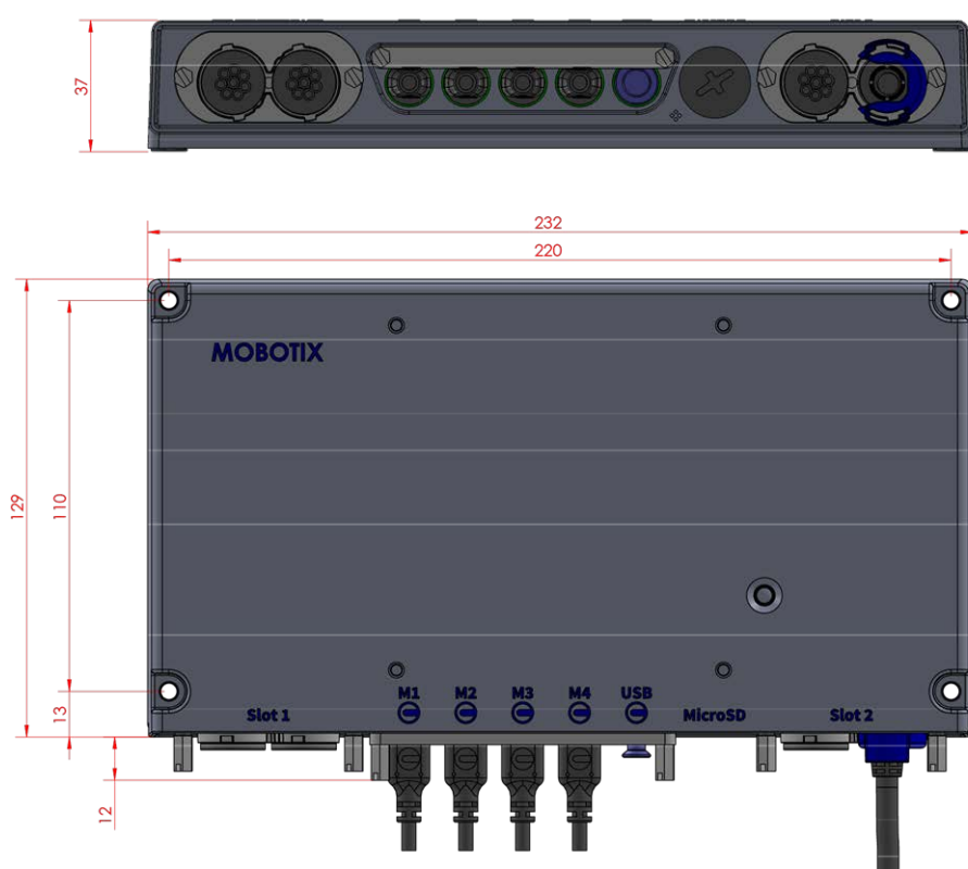
Fig. 5: S74: Tutte le misurazioni in mm
