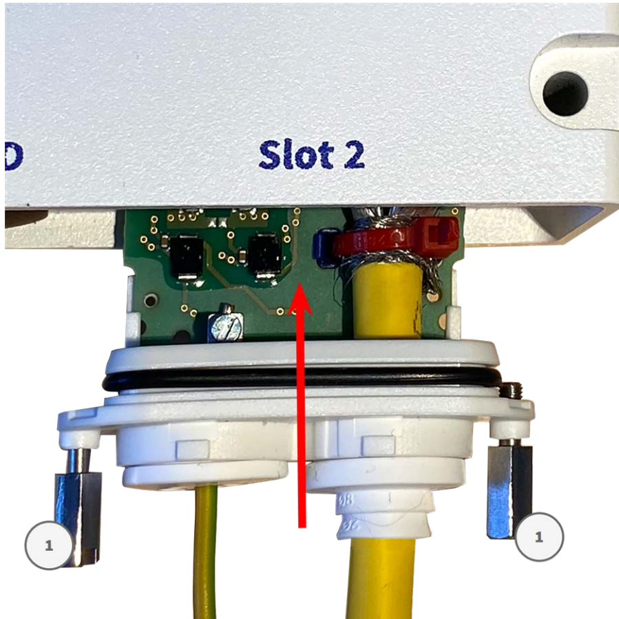
Fig. 30: Collegamento della Scheda di interfaccia LSA
