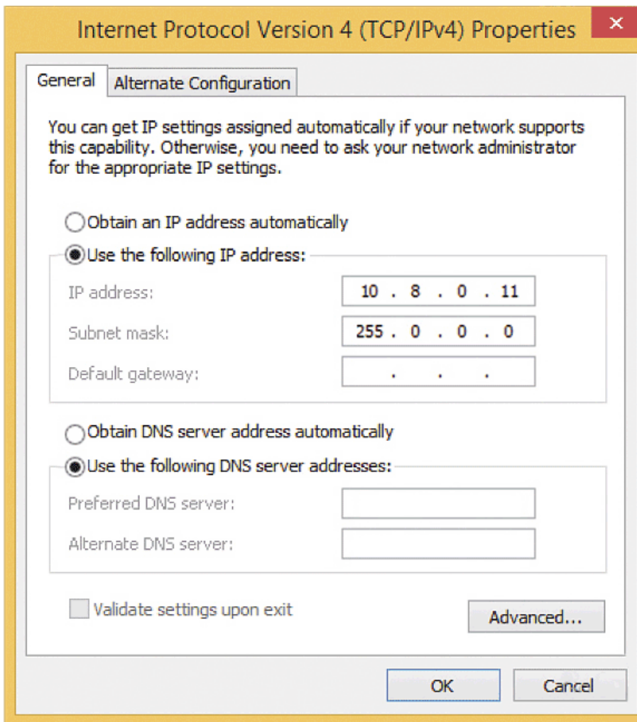
Fig. 38: Proprietà del protocollo Internet V4
