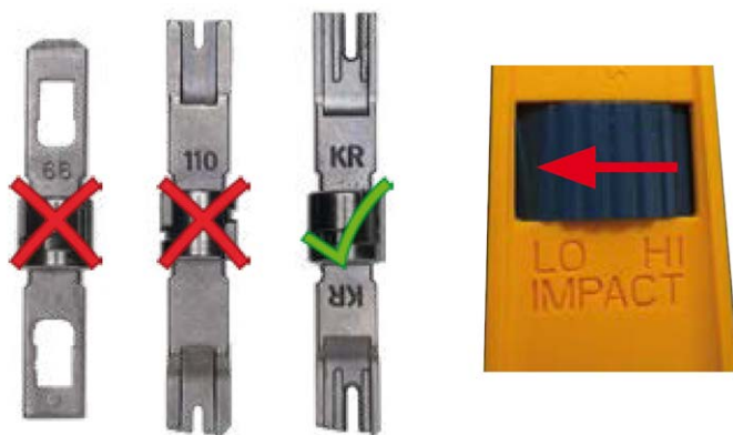
Fig. 25: Strumento LSA+/Krone impostato su impatto LOW (basso)
