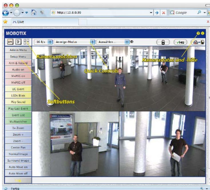
Fig. 1: Interfaccia del software della telecamera
