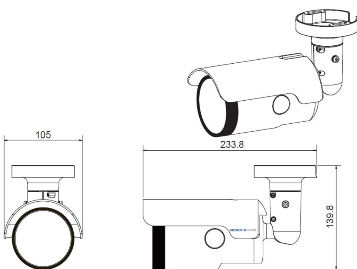
図1: 2 MP耐衝撃バレット解析カメラ: すべての測定値の単位はmm
