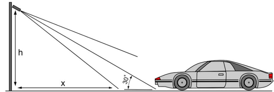
Fig. 12: Vertikale Ausrichtung der Kamera
