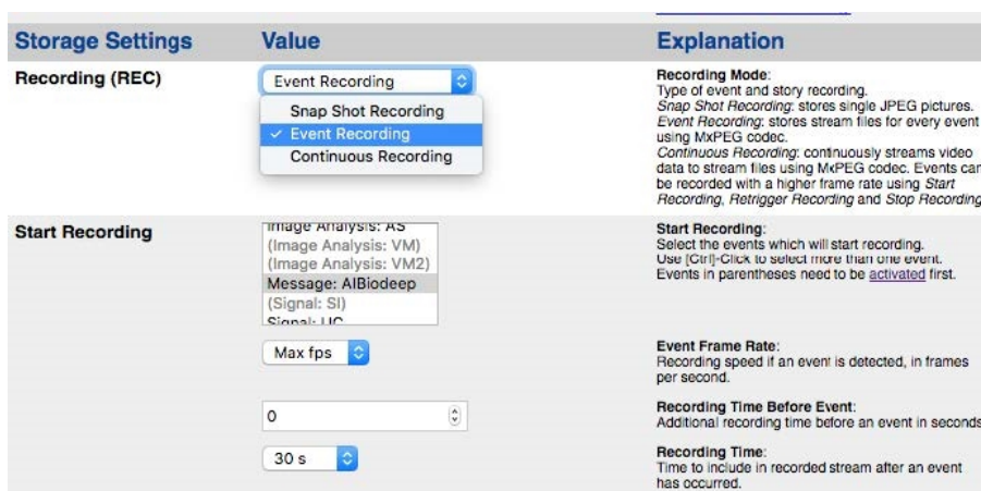
Fig. 31: Konfiguration der Aufnahmeeinstellungen der Kamera
