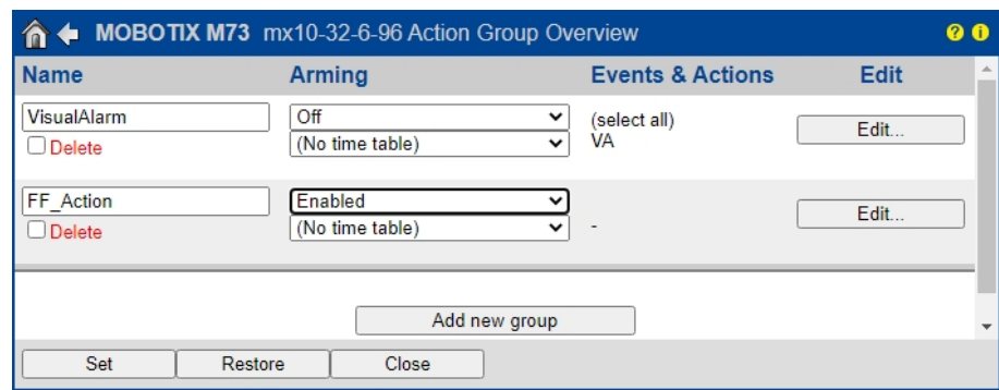
Fig. 28: Définir des groupes d'actions
