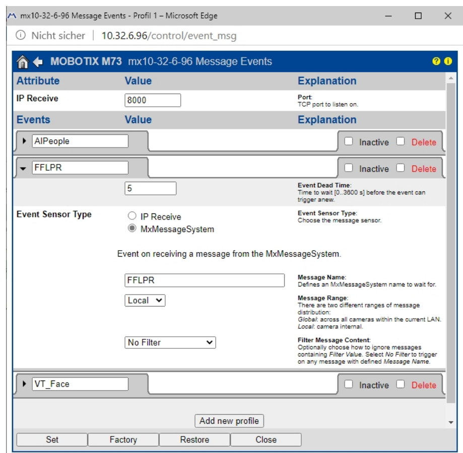
Fig. 27: Exemple : Événement de message générique de FF Group License Plate Recognition App - Region EUCA
