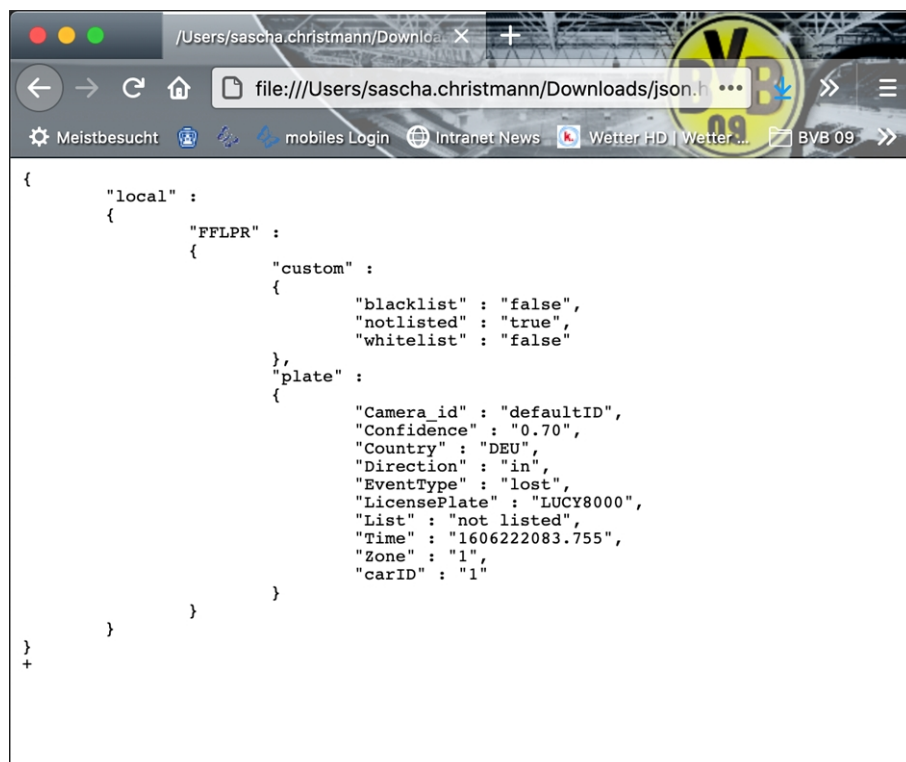
Fig. 32: Exemple : Métadonnées transmises dans un message MxMessage de FF Group License Plate Recognition App - Region EUCA
