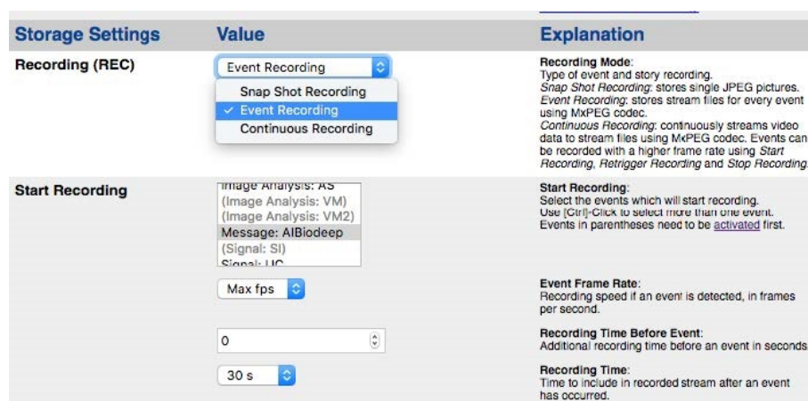
Fig. 31: Configuration des paramètres d'enregistrement de la caméra
