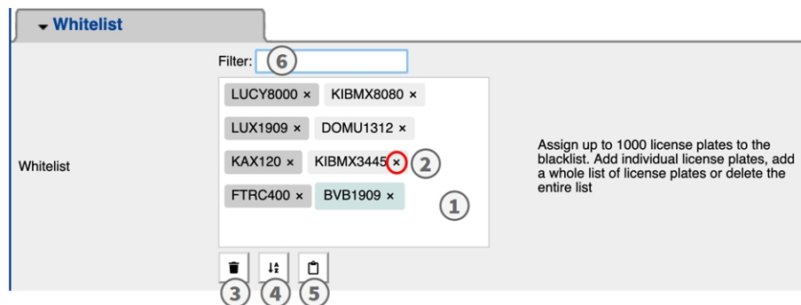
Fig. 24: Lista bianca e lista nera
