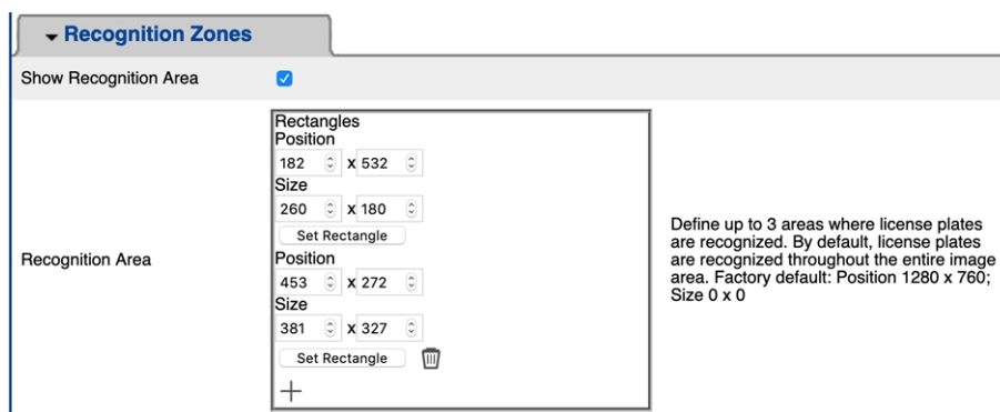
Fig. 22: Scheda "Recognition Areas" (Aree di riconoscimento)
