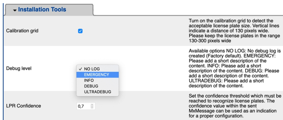
Fig. 25: Scheda "Installation Tools" (Strumenti di installazione)
