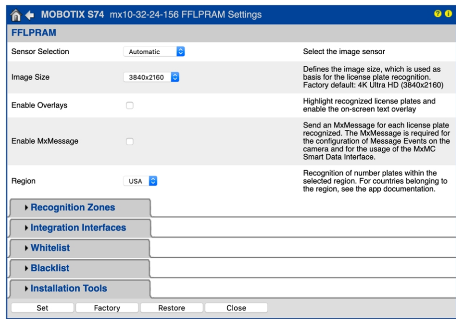
Fig. 21: Default operating mode (modalità di funzionamento predefinita): Rilevamento
