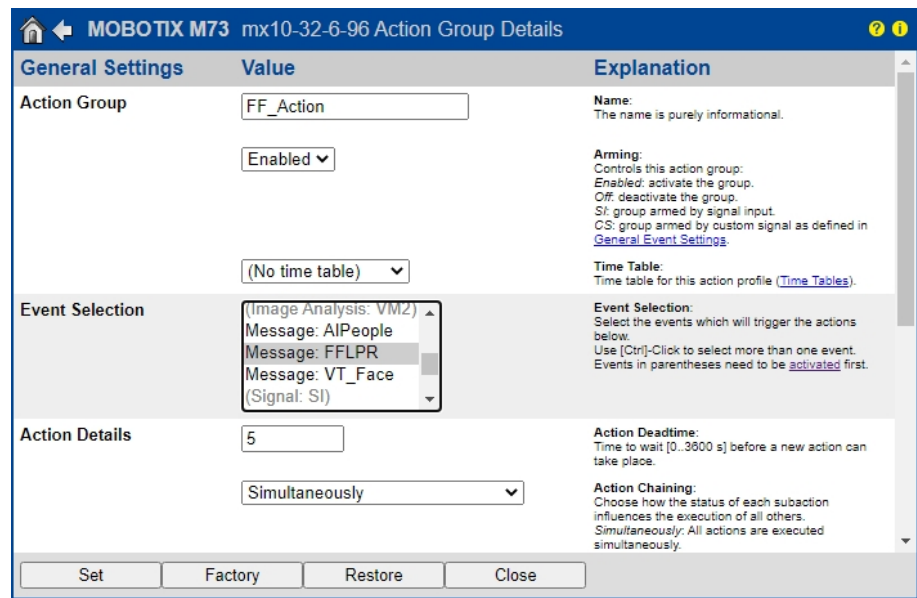
Fig. 29: Configurazione di un gruppo di azioni
