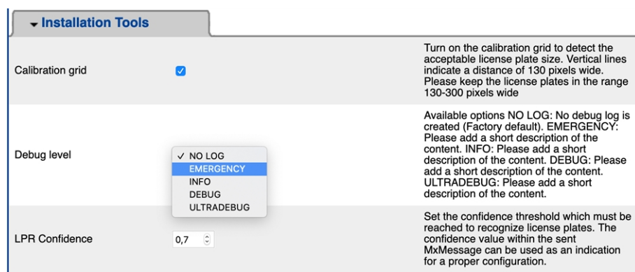
Fig. 23: Outils d'installation
