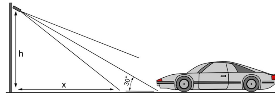
Fig. 10: Pointage vertical de la caméra
