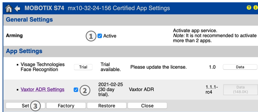
Fig. 12: Aktivierung zertifizierter Apps
