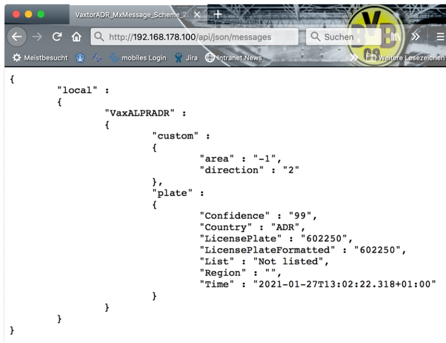
Fig. 27: Esempio: metadati trasmessi all'interno di un MxMessage dell'applicazione Vaxtor License Plate Recognition / Dangerous Goods App
