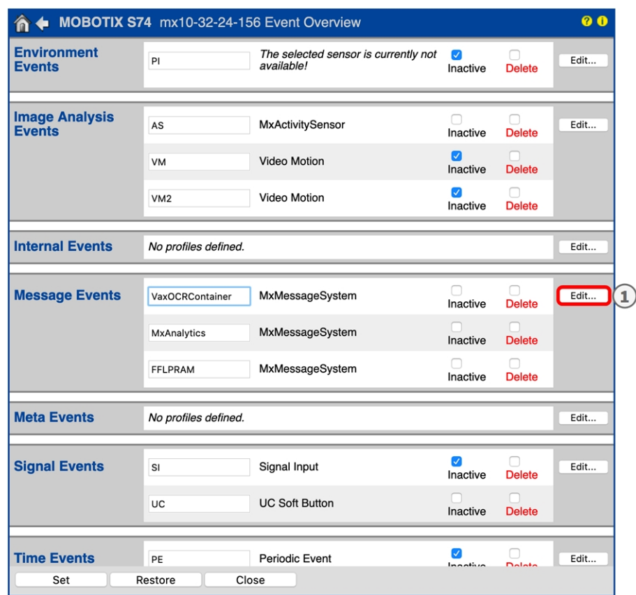
Fig. 20: Esempio: evento messaggio generico da Vaxtor Container Code Recognition App
