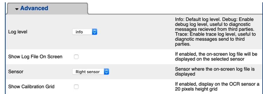
Fig. 21: Installationswerkzeuge
