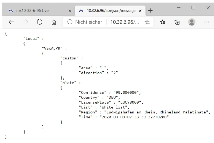
Fig. 29: Esempio: metadati trasmessi all'interno di un MxMessage dell'applicazione Vaxtor License Plate Recognition / Dangerous Goods App
