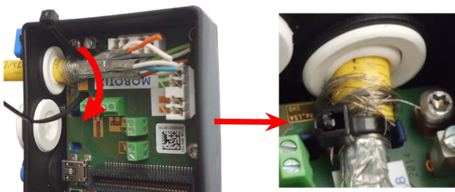
Fig. 61: Brida introducida debajo del cable de red
