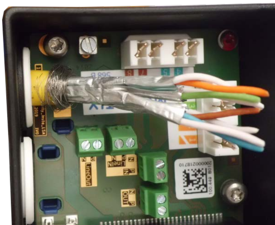
Fig. 60: El cable de red está introducido y el tapón, correctamente colocado
