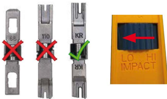
Fig. 62: Herramienta LSA+/Krone ajustada a un impacto BAJO
