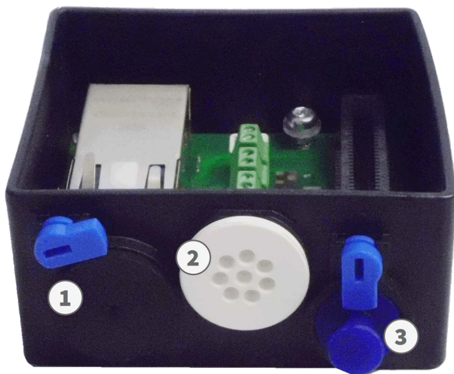
Fig. 53: Connector Box RJ45 con tapón de caucho negro C.3 ① , tapón de caucho de un solo cable C.4 ② , tapón para USB ① y dos cierres azules
