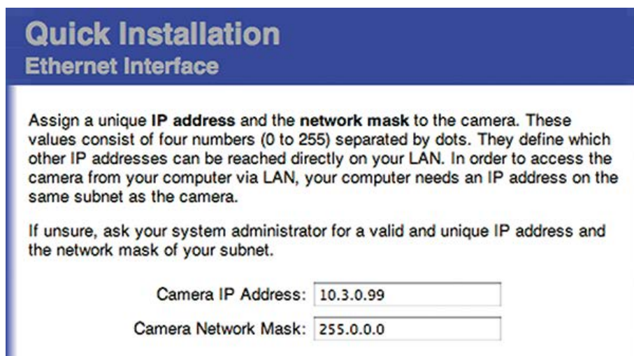
Fig. 78: Configuración de red en la interfaz web de la cámara
