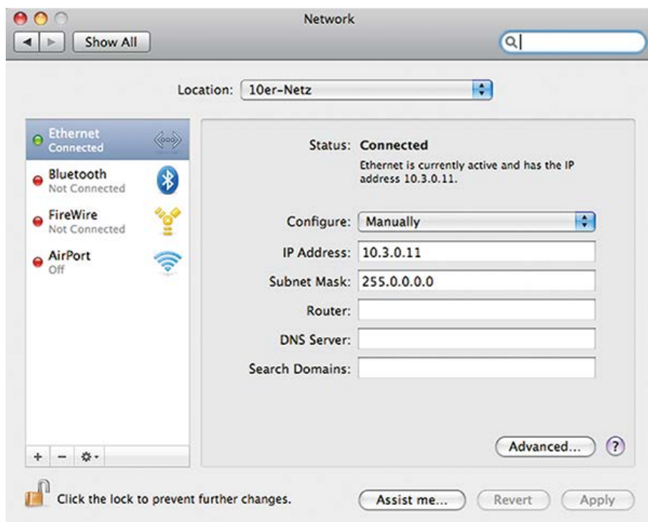
Fig. 77: Configuración de red en equipos MacOS
