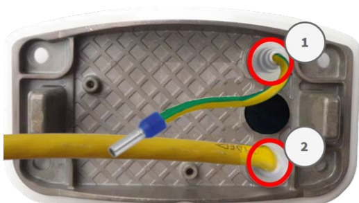
Fig. 49: Placa de montaje con cable de tierra y cable de red
