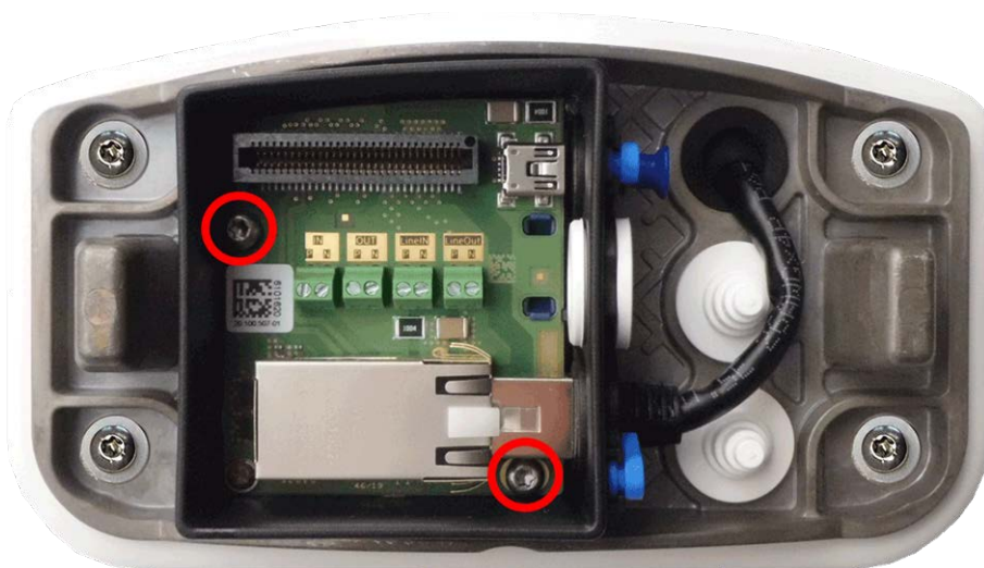
Fig. 55: Monte el Connector Box RJ45 (imagen superior) con los dos tornillos (resaltados en rojo) en la placa de montaje
