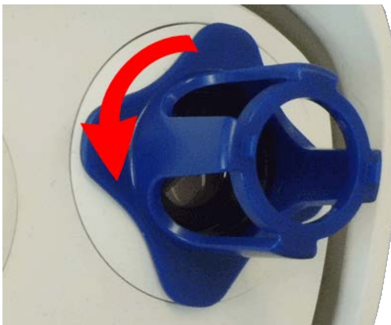
Fig. 82: Tournez le module de capteur à fond dans le sens inverse des aiguilles d'une montre
