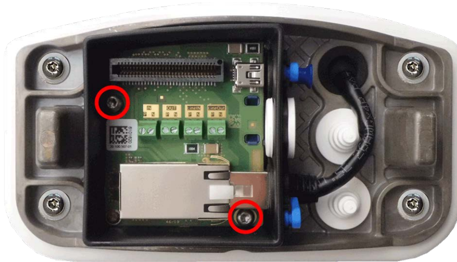
Fig. 55: Montez le Connector Box RJ45 (vue de dessus) à l'aide des deux vis (surlignées en rouge sur la figure) sur la plaque de montage
