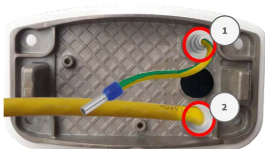
Fig. 49: Plaque de montage avec fil de terre et câble réseau
