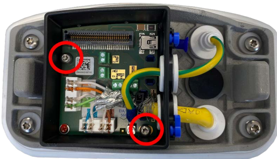
Fig. 67: Montez le Connector Box LSA (vue de dessus) à l'aide des deux vis (surlignées en rouge sur la figure) sur la plaque de montage
