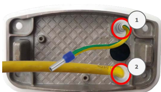
Fig. 35: Plaque de montage avec fil de terre et câble réseau
