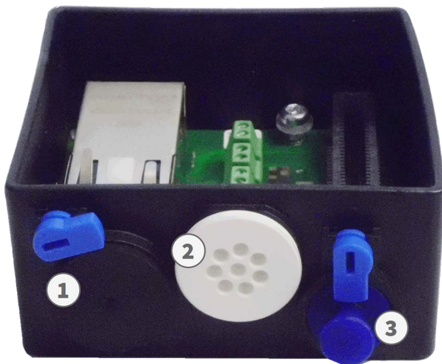
Fig. 53: Connector Box RJ45 avec bouchon en caoutchouc noir C.3 ①, bouchon en caoutchouc à un fil C.4 ②, prise USB ① et deux verrous bleus
