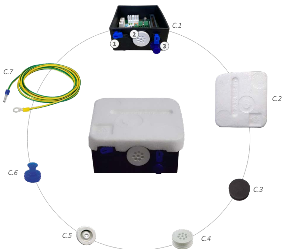
Fig. 3: Contenu de la livraison M73 Connector Box LSA
