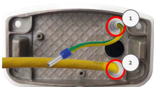
Fig. 36: Piastra di montaggio con filo di massa e cavo di rete
