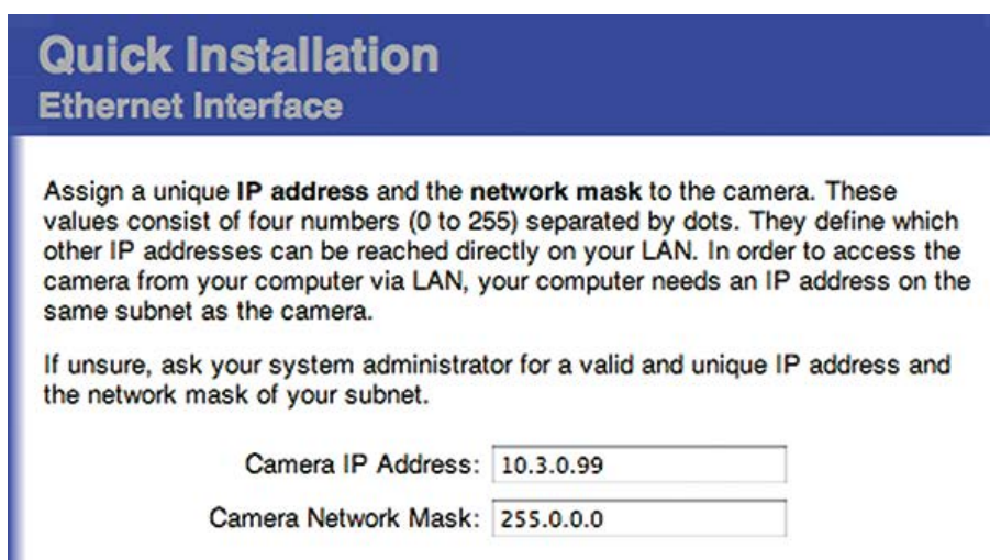
Fig. 79: Impostazioni di rete nell'interfaccia Web della telecamera.
