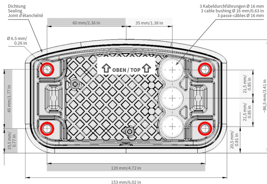
Fig. 31: Piastra di montaggio con fori per il posizionamento delle viti di fissaggio
