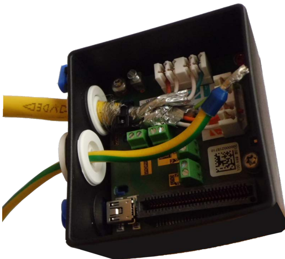
Fig. 66: Filo di massa inserito, tappo posizionato correttamente
