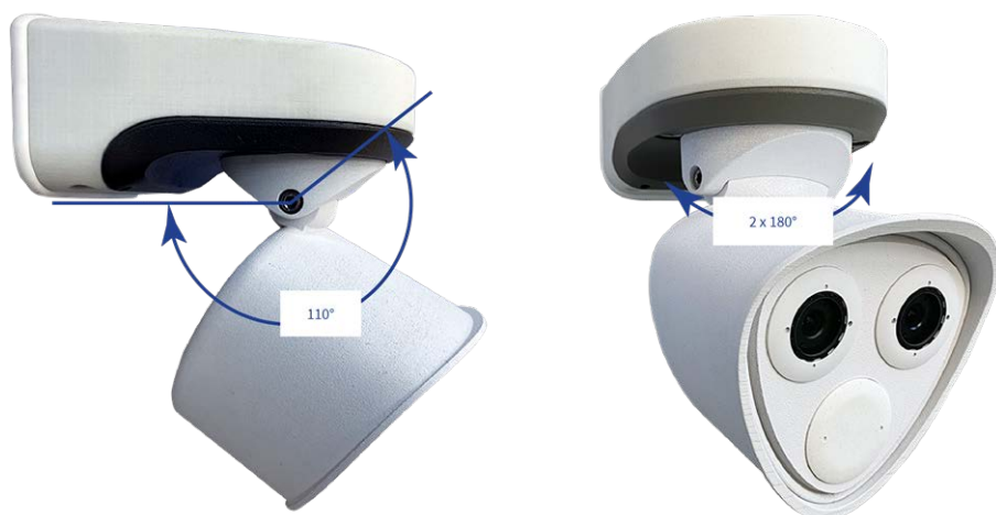
Fig. 41: Inclinazione quando montata su palo
