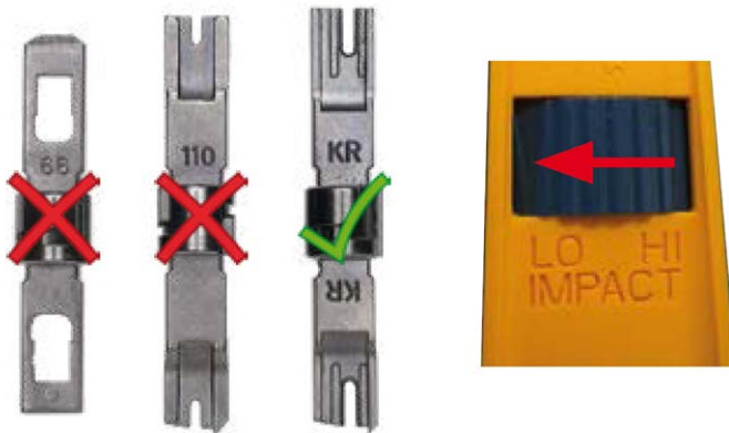
Fig. 63: Strumento LSA+/Krone impostato su impatto LOW (basso)
