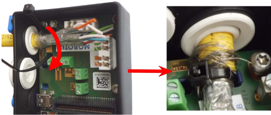
Fig. 62: Fascetta serracavi inserita sotto il cavo di rete
