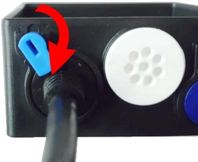
Fig. 55: Bloccare il cavo di rete nella scatola dei connettori
