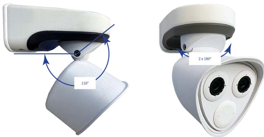
Fig. 30: Inclinazione quando montata a parete
