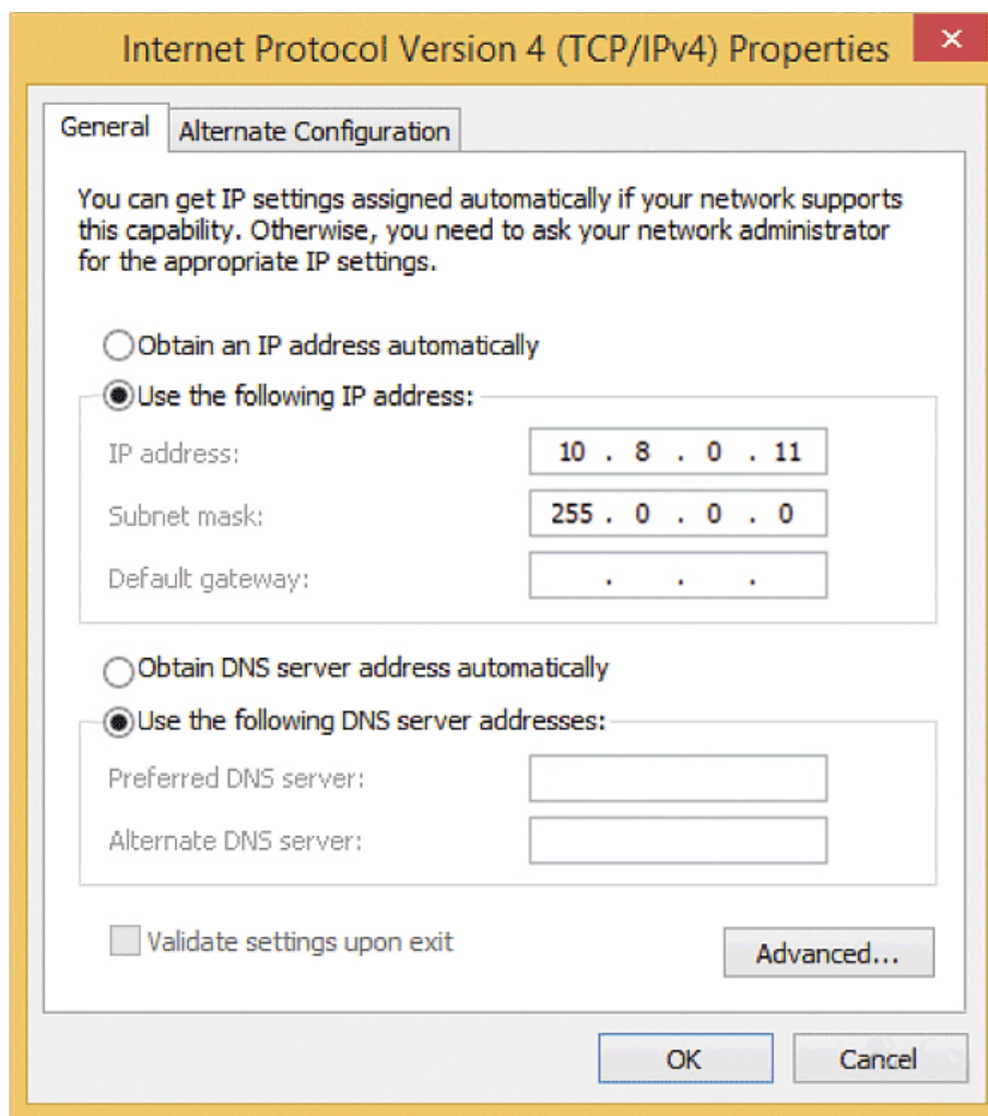
Fig. 77: Proprietà del protocollo Internet V4
