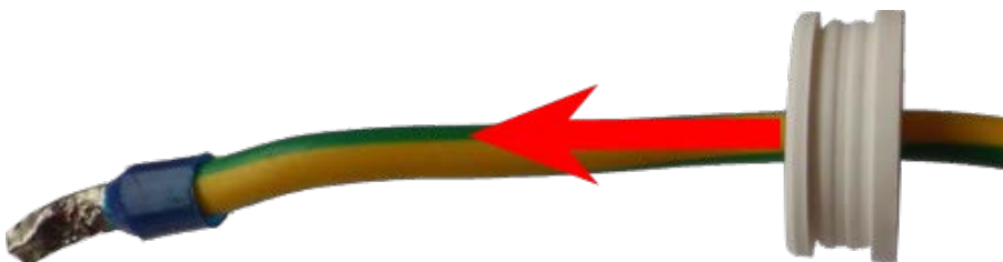
Fig. 65: Filo di massa con tappo in gomma a filo singolo C.4
