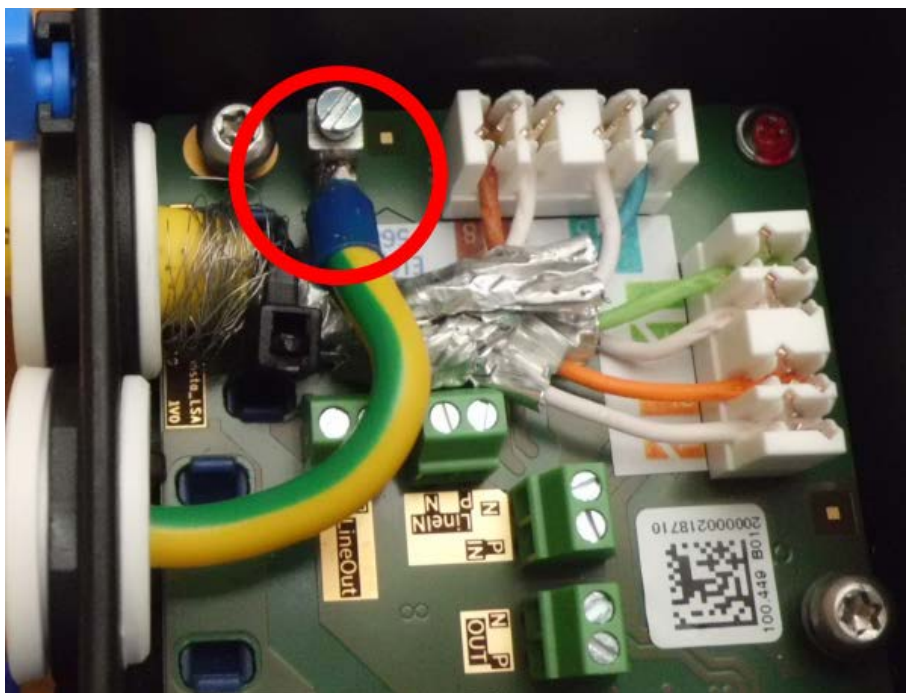
Fig. 67: Filo di massa collegato al morsetto
