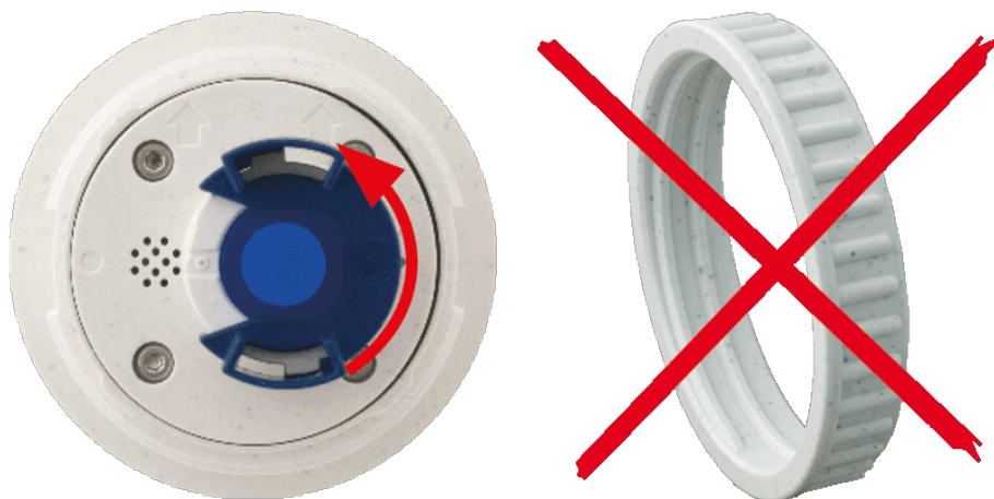
Fig. 25: Preparare il modulo sensore per il montaggio; rimuovere il dado in plastica!
