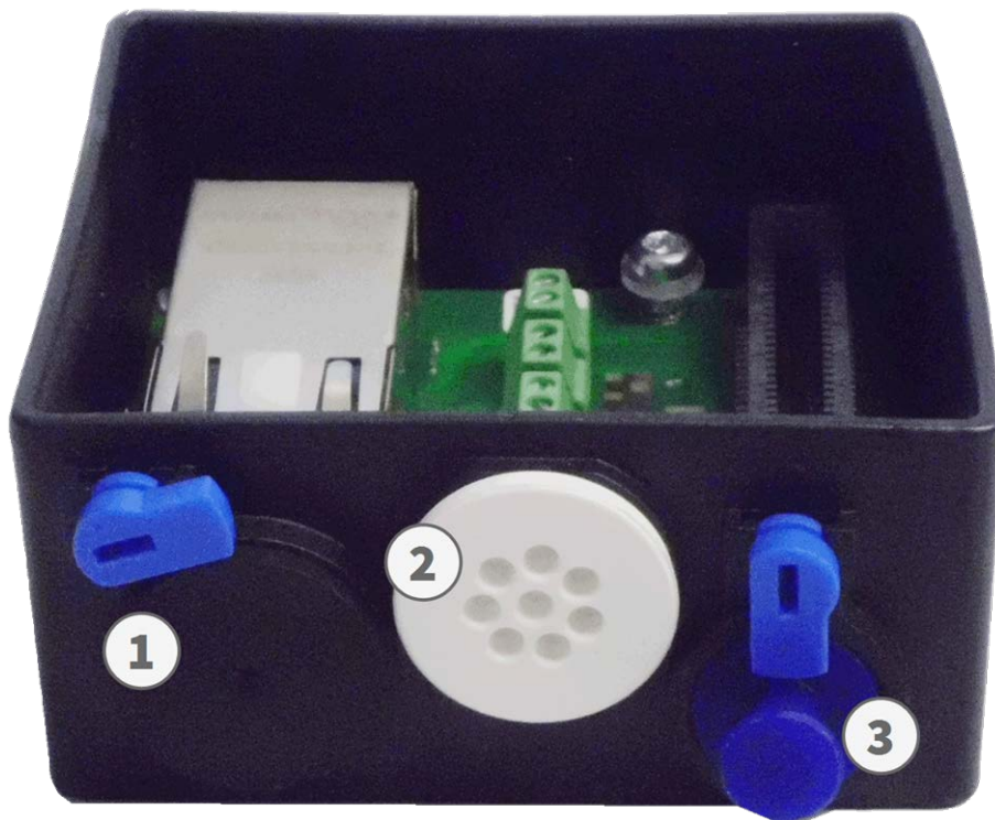
Fig. 54: Connector Box RJ45 con tappo in gomma nero C.3 ① , tappo in gomma a filo singolo C.4 ② , tappo USB ③ e due fermi blu
