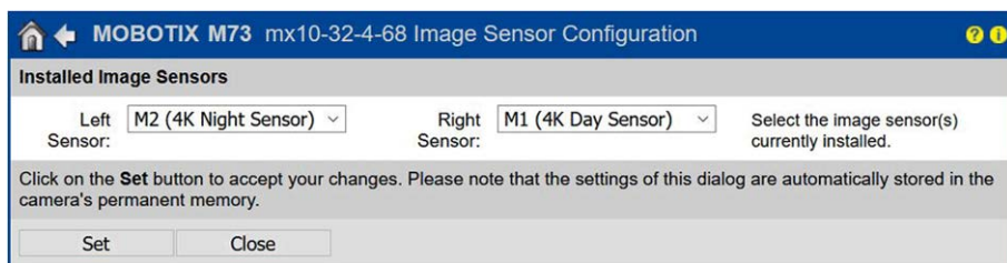
Fig. 51: Configuración de los módulos del sensor
