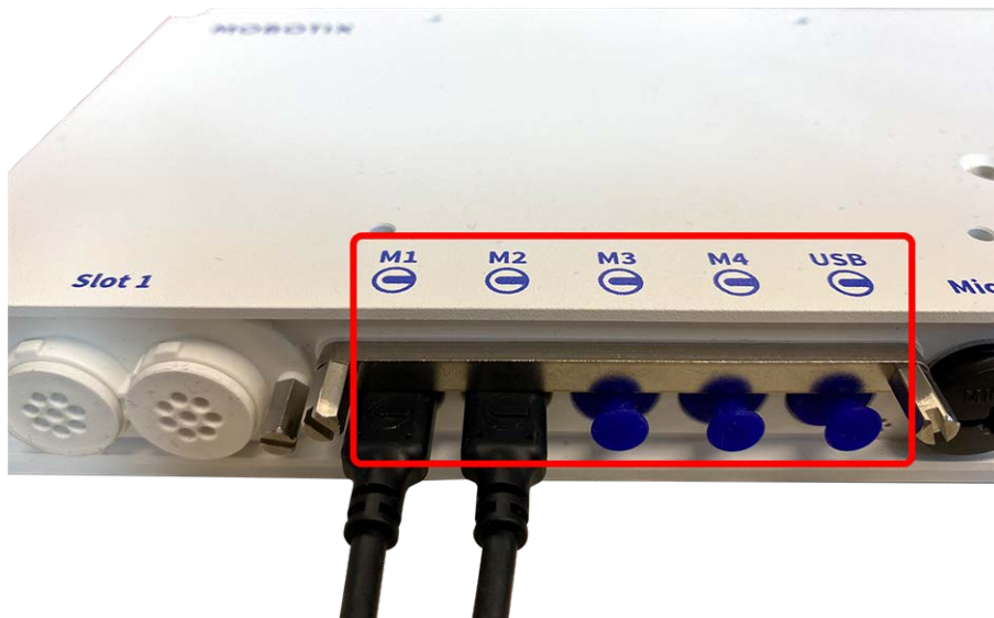
Fig. 32: 4 ports de connecteur de module et 1 interface USB-C
