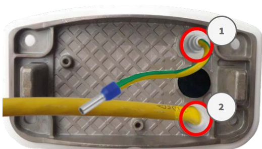
Fig. 48: Placa de montaje con cable de tierra y cable de red
