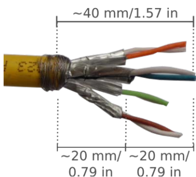
Fig. 55: Cable de red con tapón de caucho C.5
