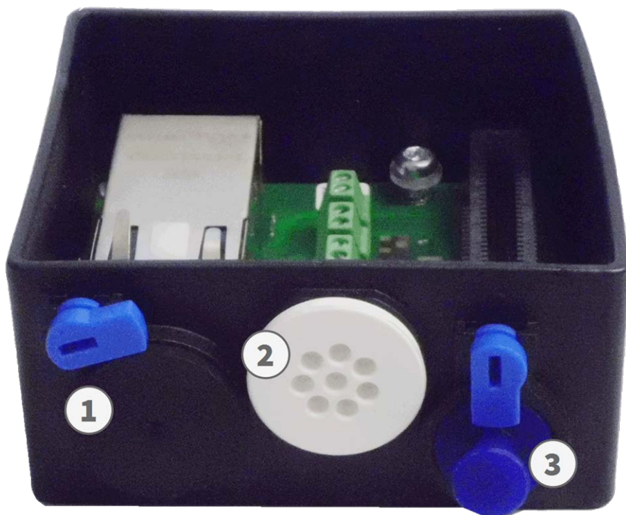
Fig. 64: Connector Box RJ45 con tapón de caucho negro C.3 ①, tapón de caucho de un solo cable C.4 ②, tapón para USB ③ y dos cierres azules
