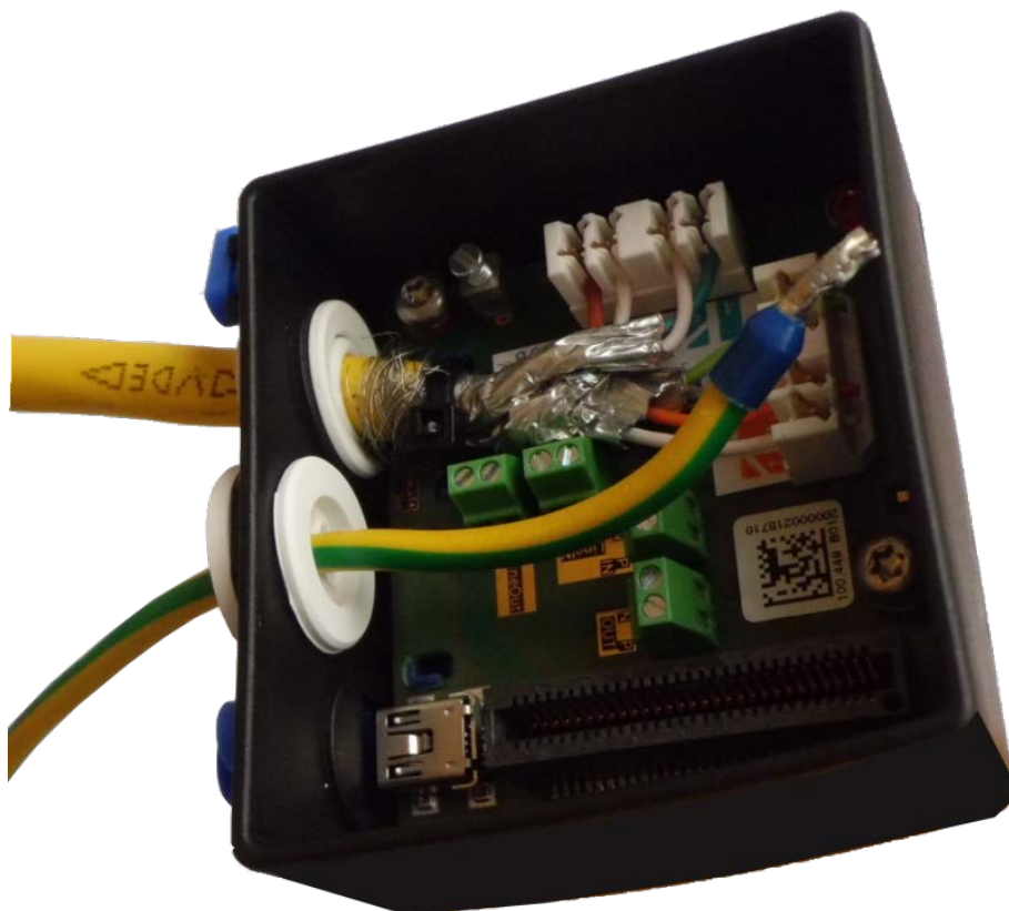
Fig. 61: El cable de tierra está introducido y tapón, correctamente colocado
