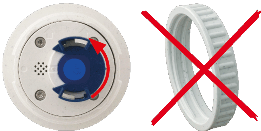
Fig. 6: Prepare el módulo de sensor para el montaje. Retire la tuerca de plástico.
