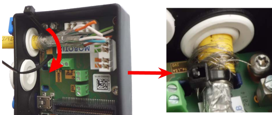
Fig. 57: Brida introducida debajo del cable de red
