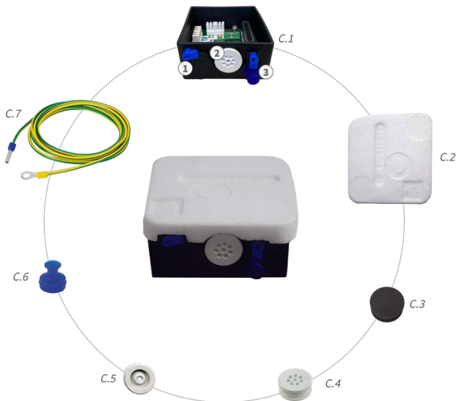
Fig. 3: Alcance de la entrega M73 Connector Box LSA
