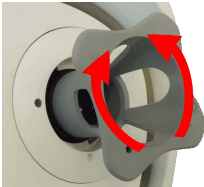
Fig. 82: Ajuste el enfoque del objetivo
