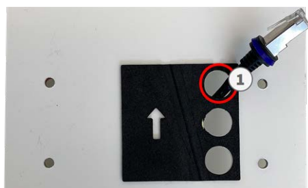
Fig. 43: Preparación de Connector Box RJ45
