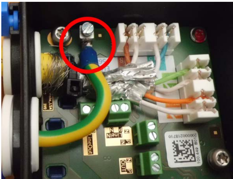
Fig. 62: Cable de tierra conectado al borne
