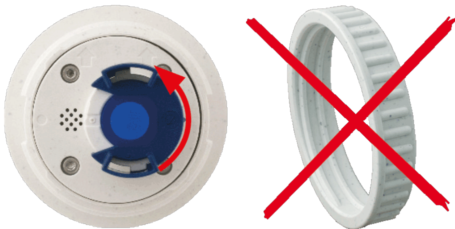
Fig. 24: Prepare el módulo de sensor para el montaje. Retire la tuerca de plástico.
