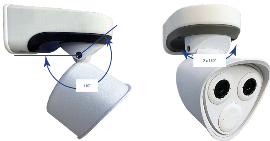
Fig. 29: Capacidad de inclinación cuando se monta en la pared
