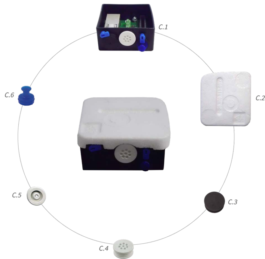
Fig. 2: Alcance de la entrega M73 Connector Box RJ45
