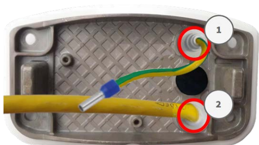
Fig. 48: Plaque de montage avec fil de terre et câble réseau
