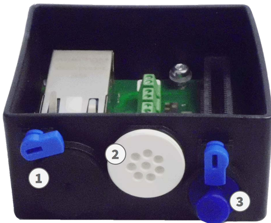
Fig. 64: Connector Box RJ45 avec bouchon en caoutchouc noir C.3 ①, bouchon en caoutchouc à un fil C.4 ②, prise USB ③ et deux verrous bleus
