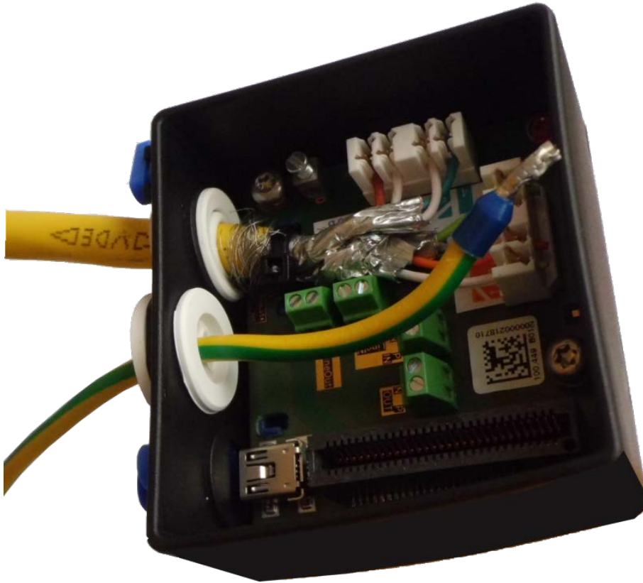
Fig. 61: Fil de terre inséré, bouchon correctement installé
