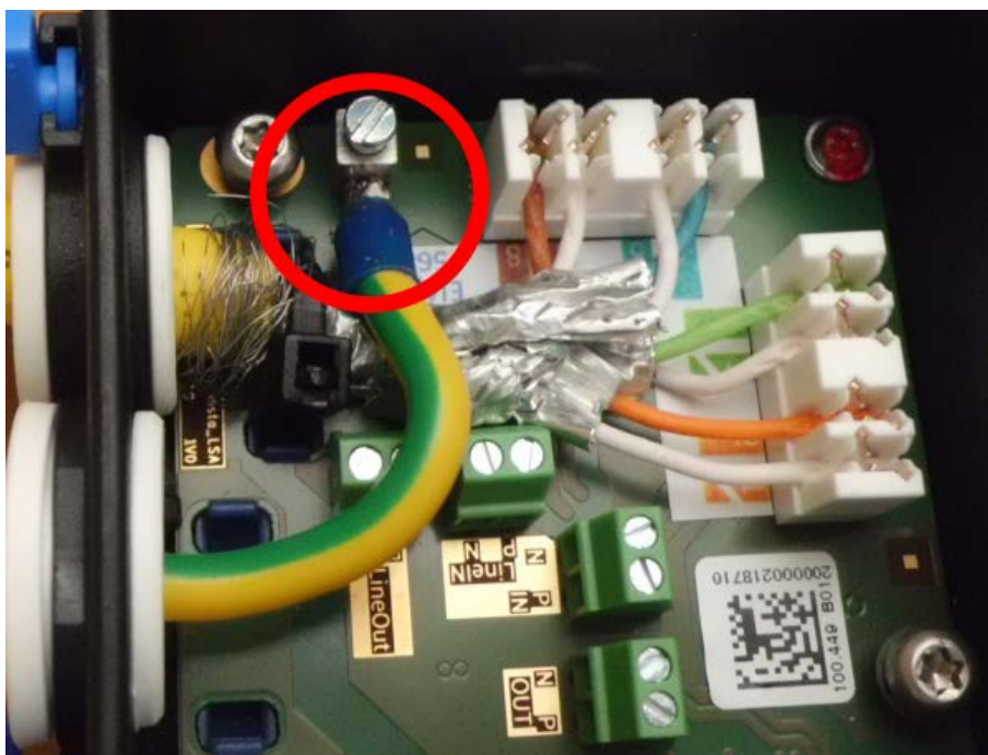
Fig. 62: Fil de terre connecté à la borne
