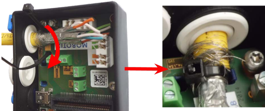
Fig. 57: Serre-câble inséré sous le câble réseau
