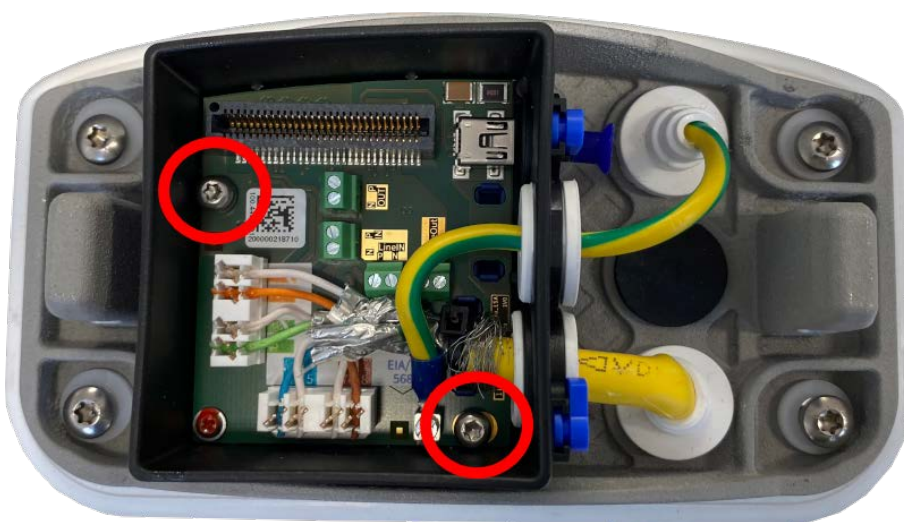
Fig. 63: Montez le Connector Box LSA (vue de dessus) à l'aide des deux vis (surlignées en rouge sur la figure) sur la plaque de montage
