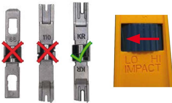
Fig. 58: Outil LSA+/Krone défini sur un impact LOW (Faible)
