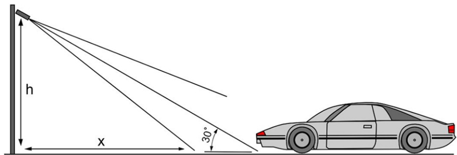
Abb. 10: Vertikale Ausrichtung der Kamera
