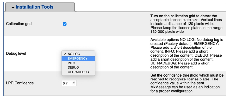
Fig. 23: Herramientas de instalación
