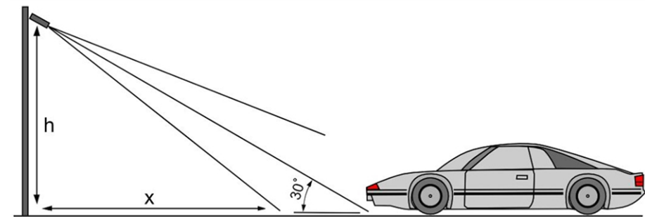
Fig. 10: Orientación vertical de la cámara
