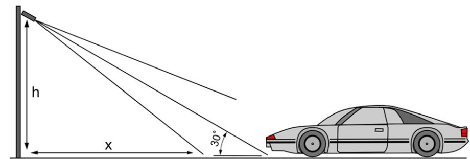
Fig. 10: Puntamento verticale della telecamera
