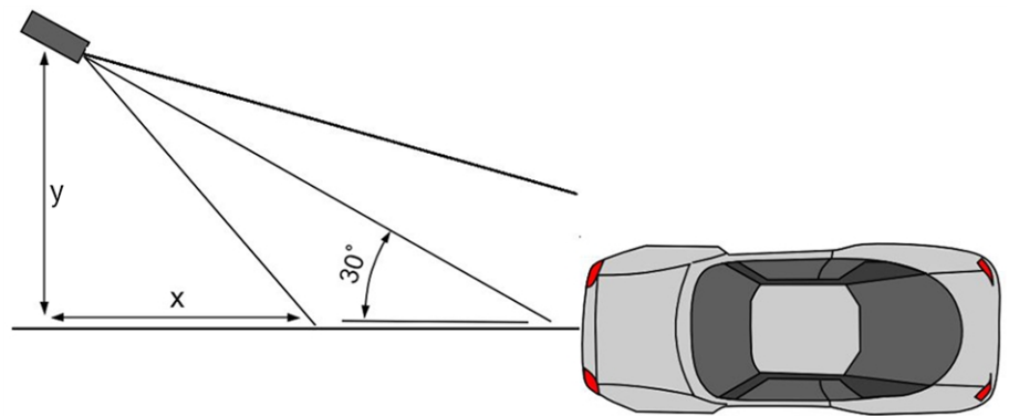
Fig. 11: Allineamento orizzontale della telecamera
