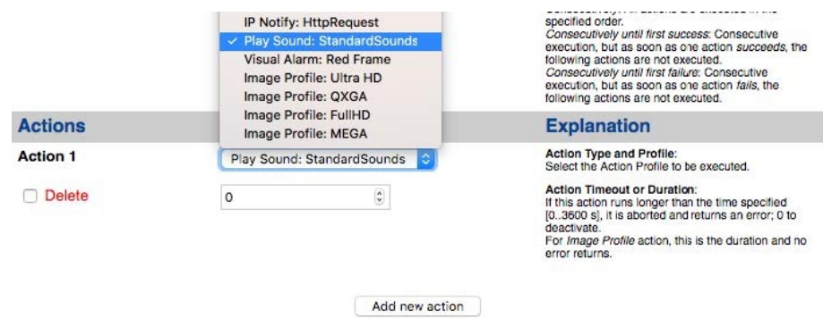
Fig. 22: Sélectionner le type et profil d'action.
