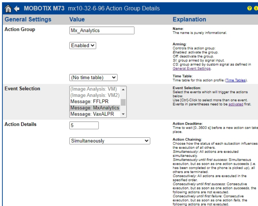
Fig. 21: Configurer un groupe d'actions
