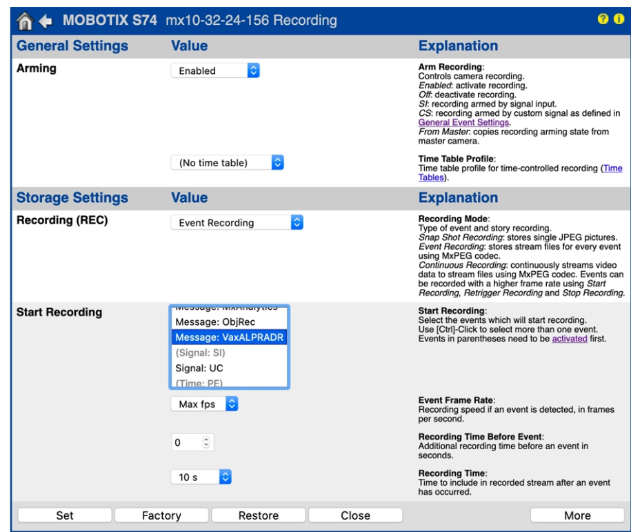
Fig. 26: Configurazione delle impostazioni di registrazione della telecamera
