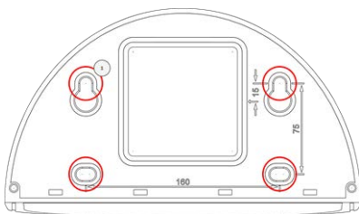
Abb. 7: Montageplatte mit Bohrungen zur Positionierung der Befestigungsschrauben
