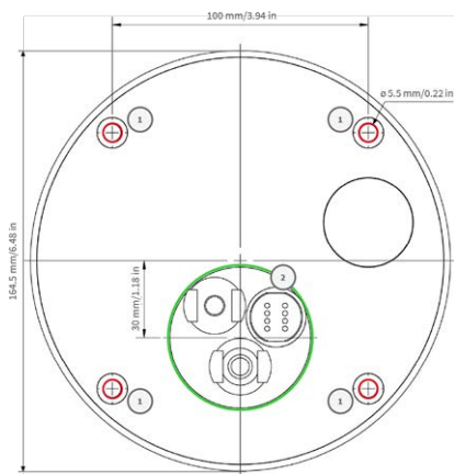
Abb. 6: Bohrschablone mit Löchern zur Positionierung der Befestigungsschrauben (rote Kreise) und für die Unterputzsteckdose (grüner Kreis)
