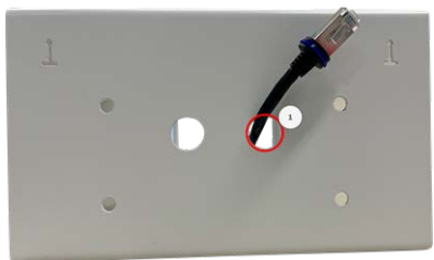
Abb. 14: Netzwerkverkabelung vorbereiten
