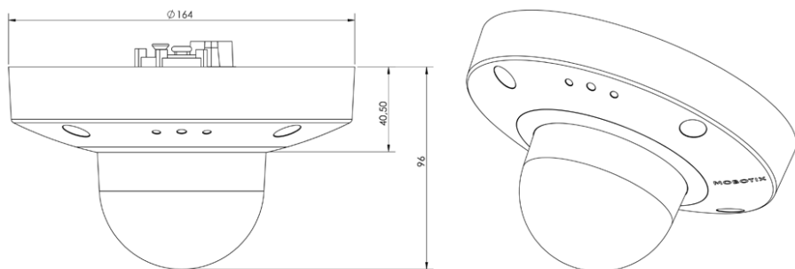
Abb. 4: D71: Alle Maßangaben in mm
