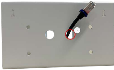
Abb. 11: Netzwerkverkabelung vorbereiten
