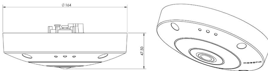
Abb. 1: Q71: Alle Maßangaben in mm
